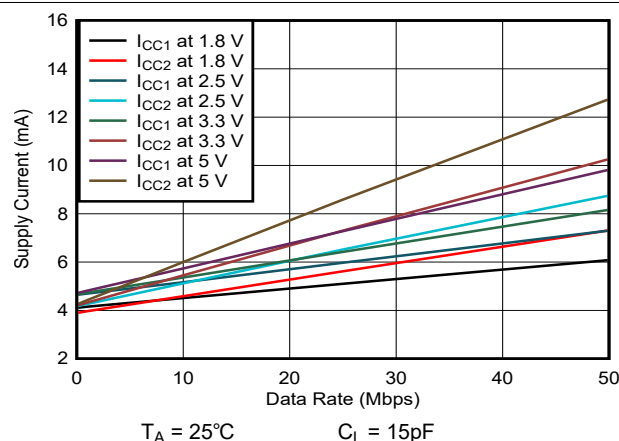
図 5-7. ISO6762-Q1 の電源電流とデータ レートとの関係 (15pF 負荷時)
