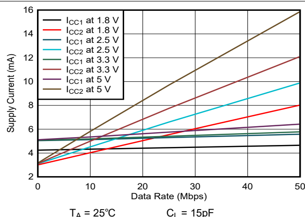
図 5-3. ISO6760-Q1 の電源電流とデータ レートとの関係 (15pF 負荷時)
