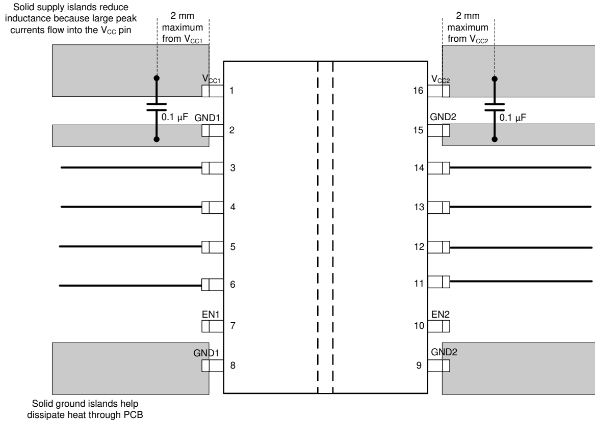
図 8-9. レイアウト例
