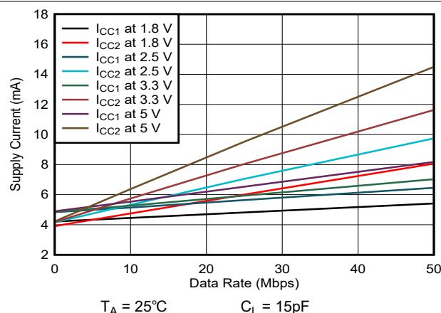
図 5-5. ISO6761-Q1 の電源電流とデータ レートとの関係 (15pF 負荷時)
