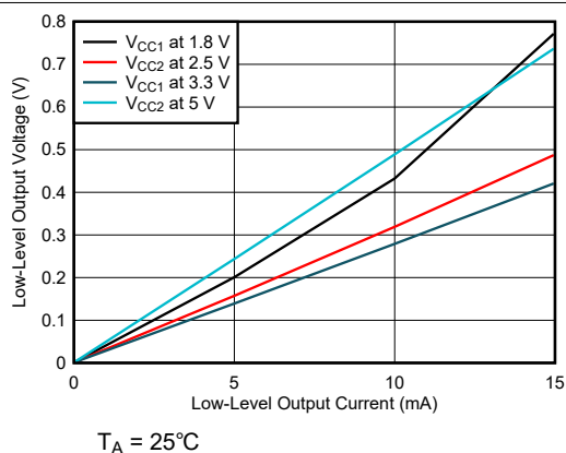
図 5-14. Low レベル出力電圧と Low レベル出力電流との関係
