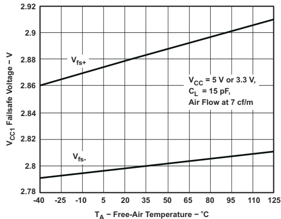
図 6-7. V_{CC1} フェイルセーフスレッシュホールド電圧と自由通気温度との関係
