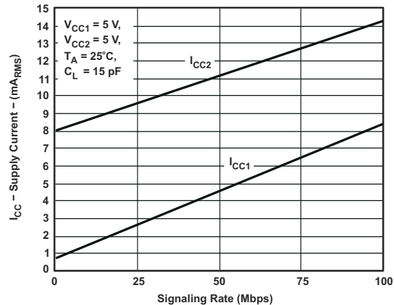
図 6-2. RMS 電源電流と信号速度との関係
