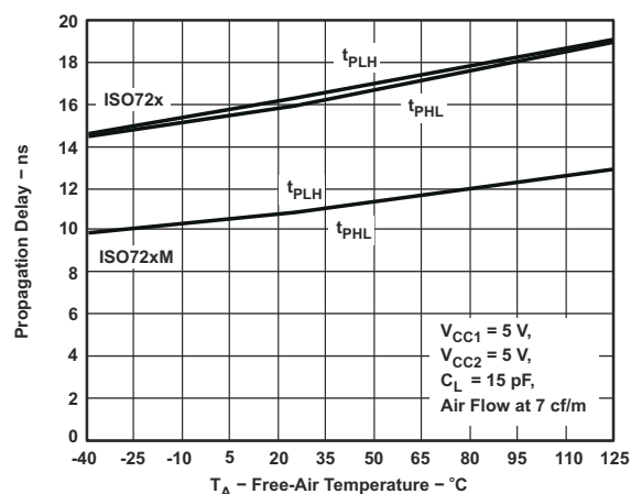
図 6-4. 伝搬遅延と自由気流温度との関係
