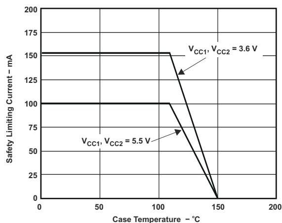
図 9-6. VDE に従う制限電流の熱特性低下曲線
