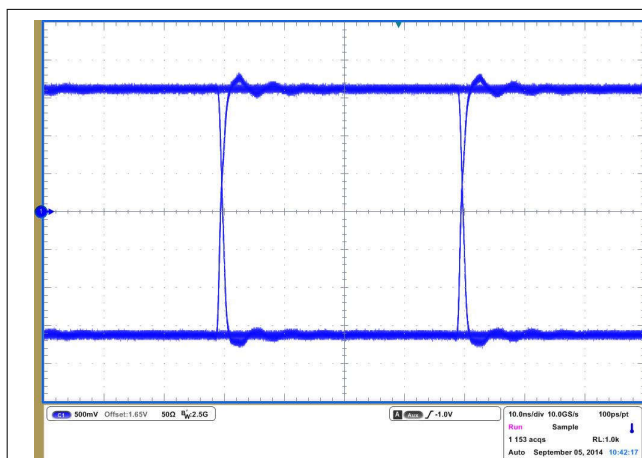
図 9-4. 25Mbps、3.3V、25°Cの ISO721M アイダイアグラム
