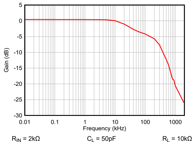
図 9-6. R_L = 10\text{k}\Omega での帯域幅
