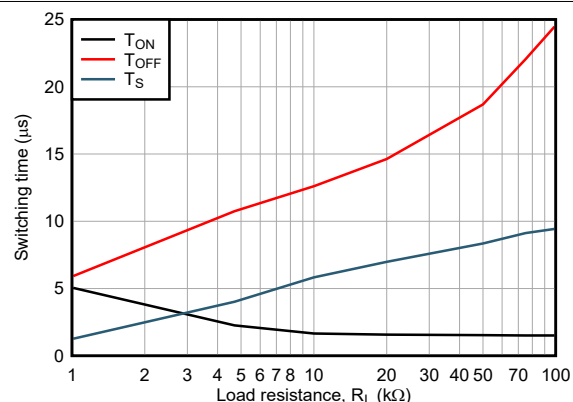
I_F = 1.6mA ISOM8112-Q1 および ISOM8117-Q1 V_{CC} = 5V
