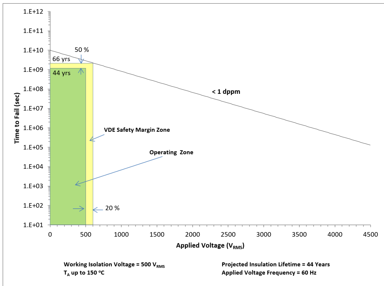
図 9-8. 絶縁寿命予測データ
