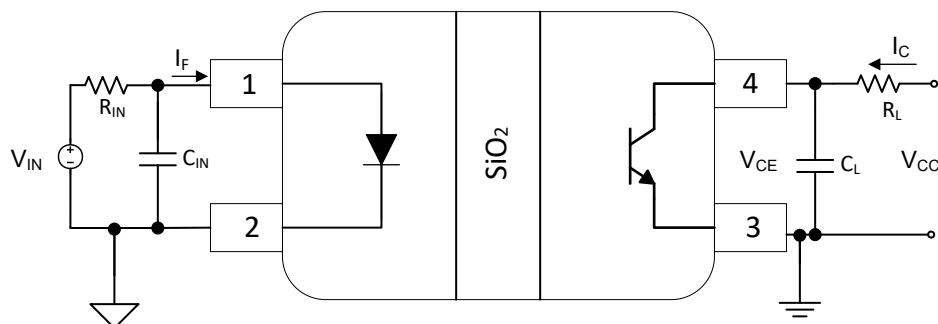
図 7-4. ISOM811[0-3]-Q1 帯域幅のテスト回路
