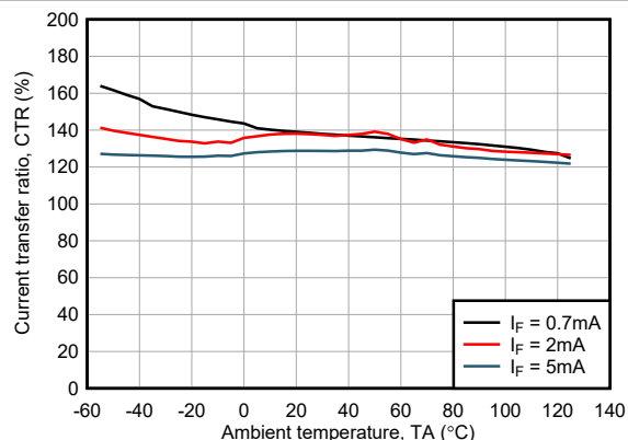
ISOM8110-Q1 および ISOM8115-Q1 V_{CE} = 5V
