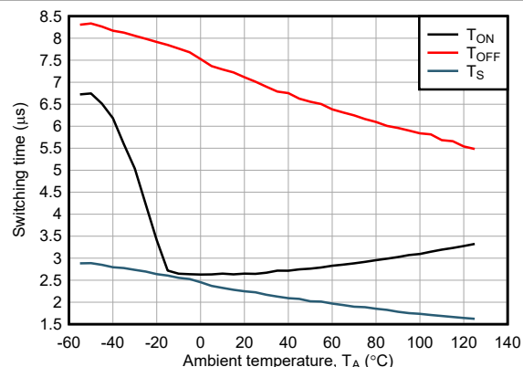
I_F = 1.6mA ISOM8110-Q1 および ISOM8115-Q1 R_L = 4.7k\Omega
