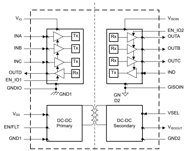
ISOW7741 概略回路図
