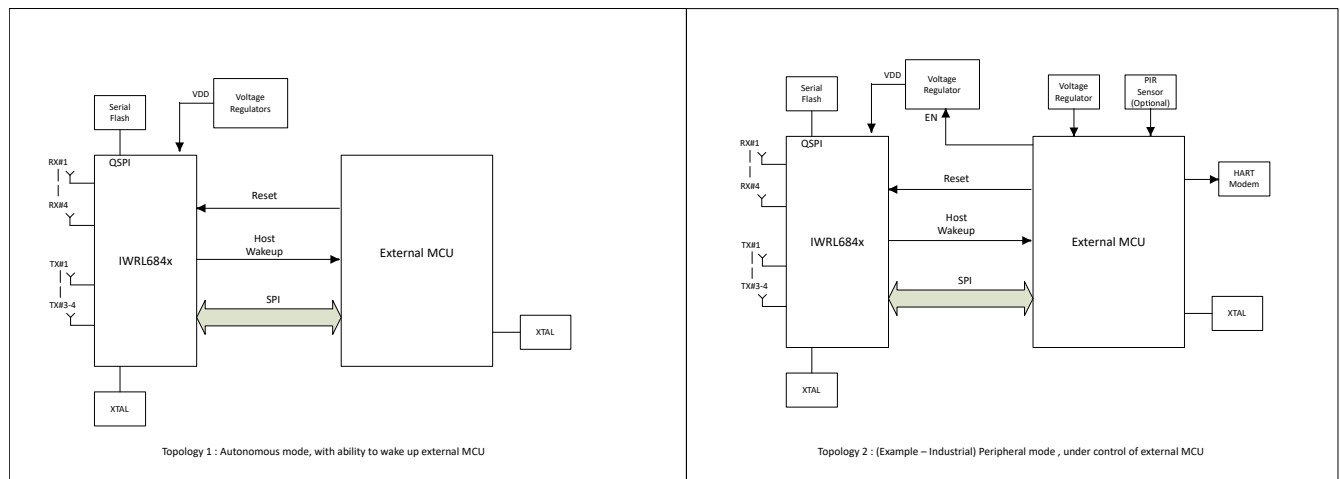
図 7-1. System Topologies
