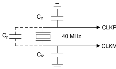
図 7-8. Crystal Implementation
