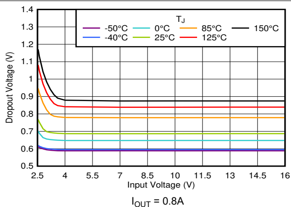
図 5-12. V_{DO} vs V_{IN}
