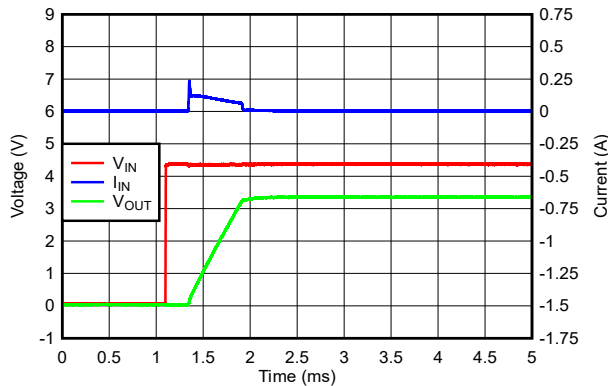
図 7-3. 22 \mu F の C_{OUT} を使用した場合のスタートアップおよび突入電流
