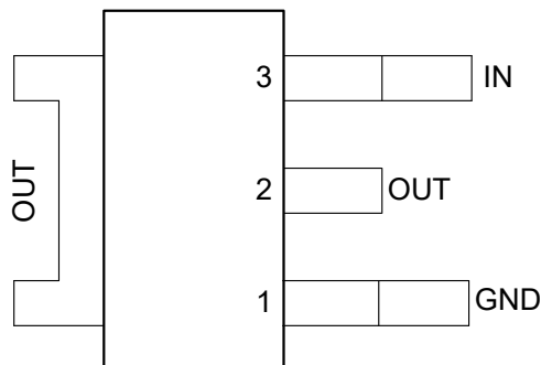
図 4-2. KVV パッケージ、3 ピン TO-252 (上面図)
