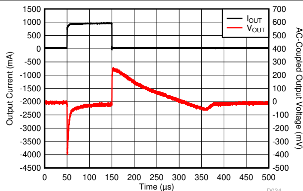
図 5-7. I_{OUT} 過渡電流 (1mA~1A)
