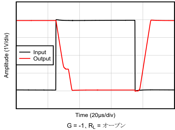
図 6-30. 大信号ステップ応答、G = -1
