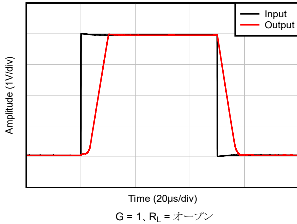
図 6-29. 大信号ステップ応答、G = 1
