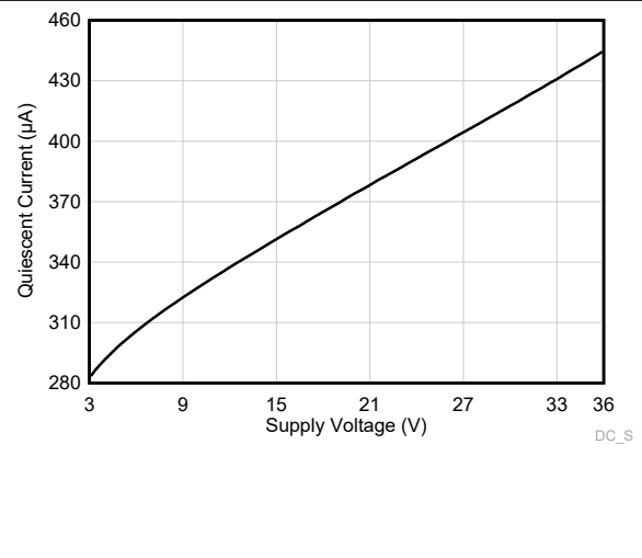
図 5-22. 静止電流と電源電圧との関係
