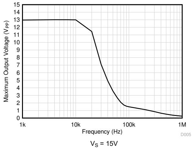
図 5-36. 最大出力電圧と周波数との関係 V_S = 15\text{V}
