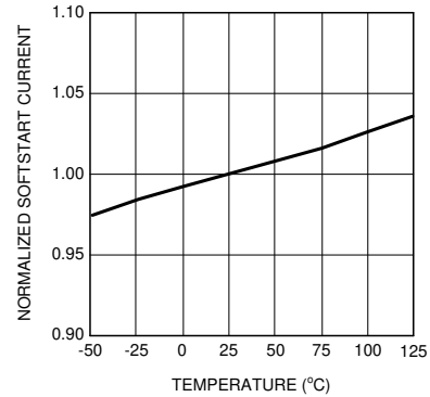
図 5-2. ソフトスタート電流と温度との関係
