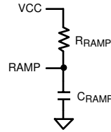
図 6-3. V_{OUT} > 7.5V の場合、 V_{CC} に対する R_{RAMP}
