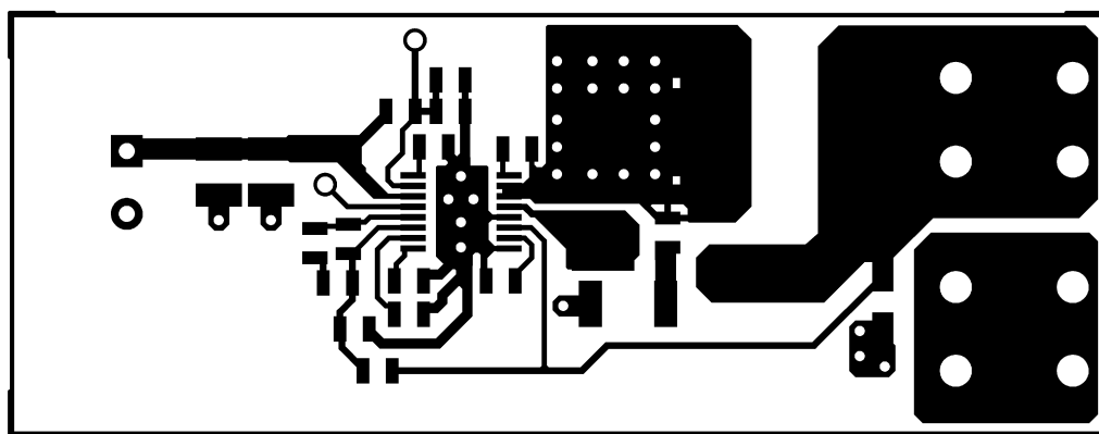
図 7-11. コンポーネント側
