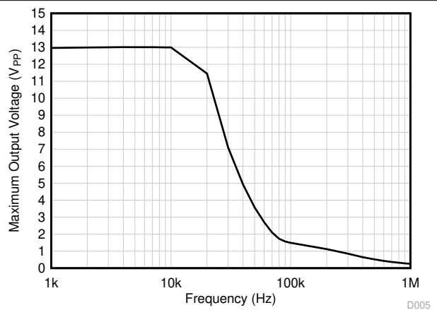
図 5-36. 最大出力電圧と周波数との関係
