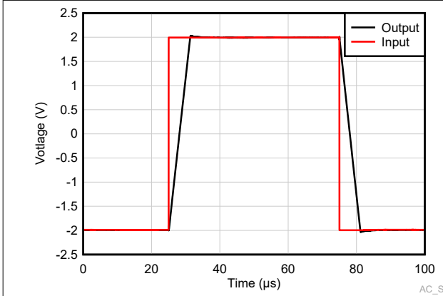
図 5-33. 大信号ステップ応答
