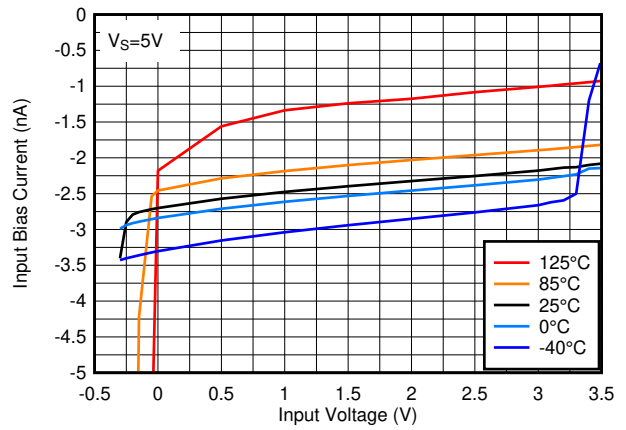
図 5-16. 入力バイアス電流と入力電圧との関係、5V
