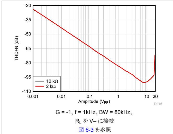
図 5-21. THD+N と出力振幅との関係、 G = -1
