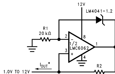
図 8-9. 高精度 1μA ~ 1mA 電流ソース
