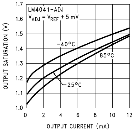
図 5-9. 出力飽和 (SOT-23 のみ)
