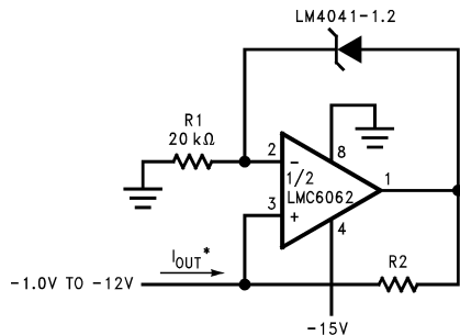
図 8-8. 高精度 1μA ~ 1mA 電流シンク
