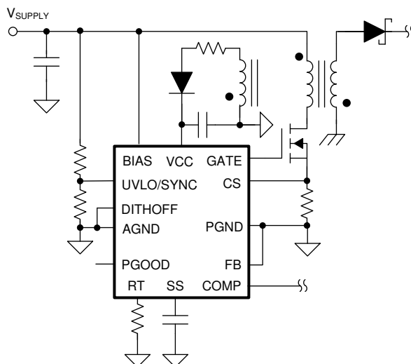
図 9-7. External VCC Supply (BIAS \geq VCC)
