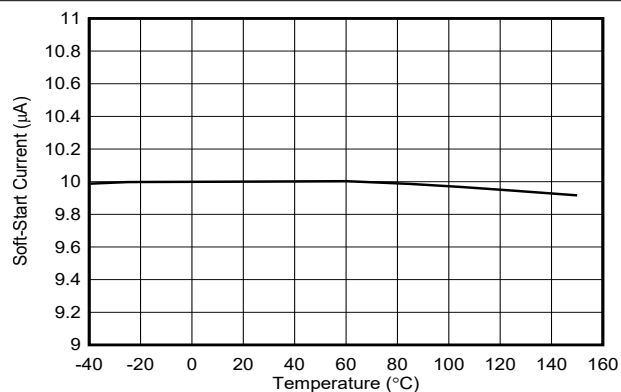
FIG 8-6. I_{SS} vs Temperature
