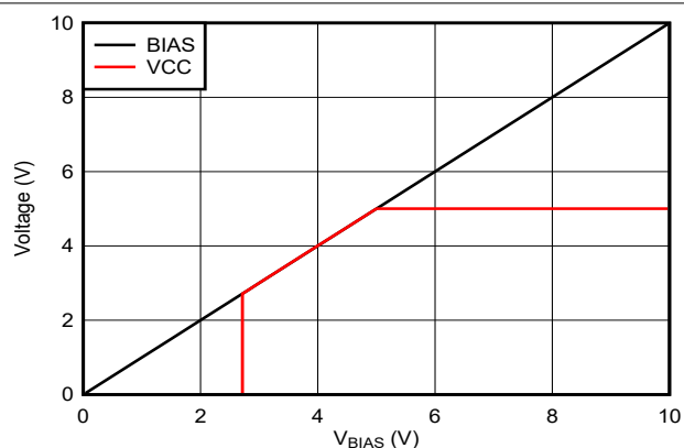
FIG 8-4. V_{VCC} vs V_{BIAS}
