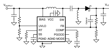
代表的な SEPIC アプリケーション
