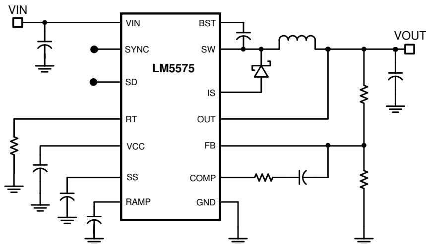
概略回路図
