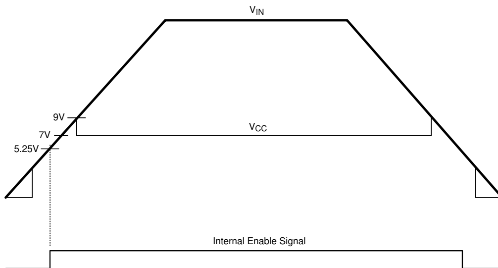
図 6-1. V IN および V CC シーケンス
