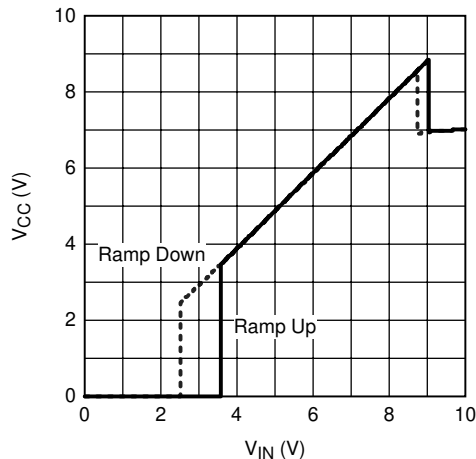
図 5-5. V_{CC} と V_{IN} R_L = 7kΩ との関係
