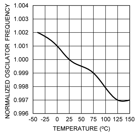
図 5-2. ( F_{OSC} = 200kHz 時)
