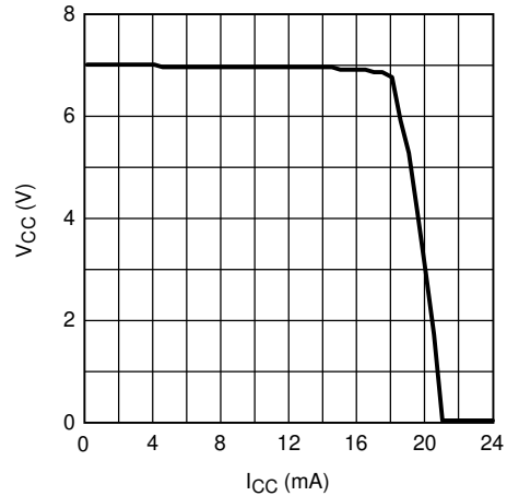
図 5-4. V_{CC} と I_{CC} V_{IN} = 12V との関係
