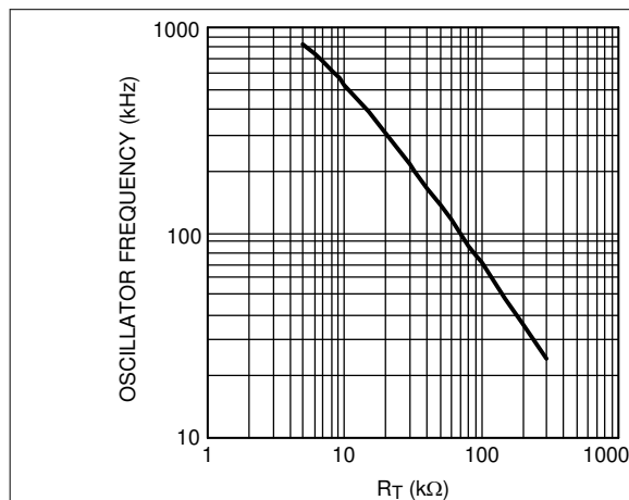
図 7-8. 発振器周波数と R_T との関係
