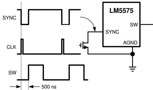
図 6-2. 外部クロックからの同期
