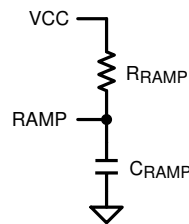
図 6-6. V OUT > 7.5V の場合、V CC に対する R RAMP
