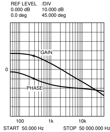
図 7-5. 変調器のゲインと位相 R = 5Ω および C = 177μF 負荷アウト
