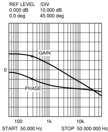
図 7-10. 変調器のゲインと位相 R = 5\Omega および C = 177\mu\text{F} 負荷アウト
