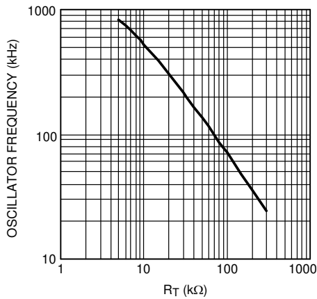
図 5-1. 発振器周波数と R_T
