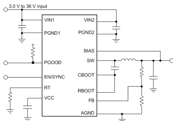
概略回路図
