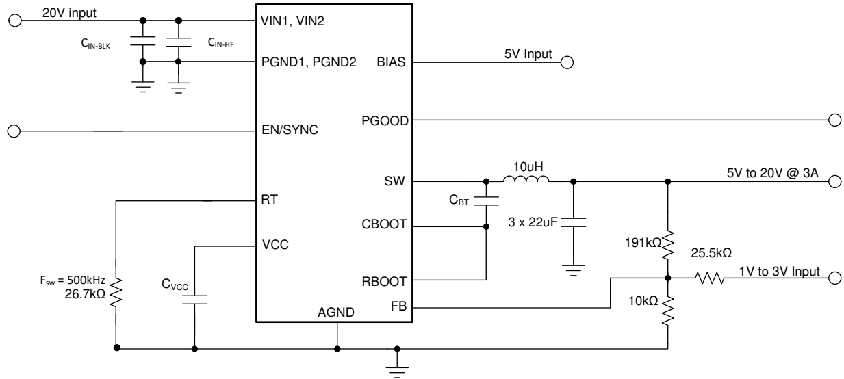
図 9-44. USB Type-C Power Supply
