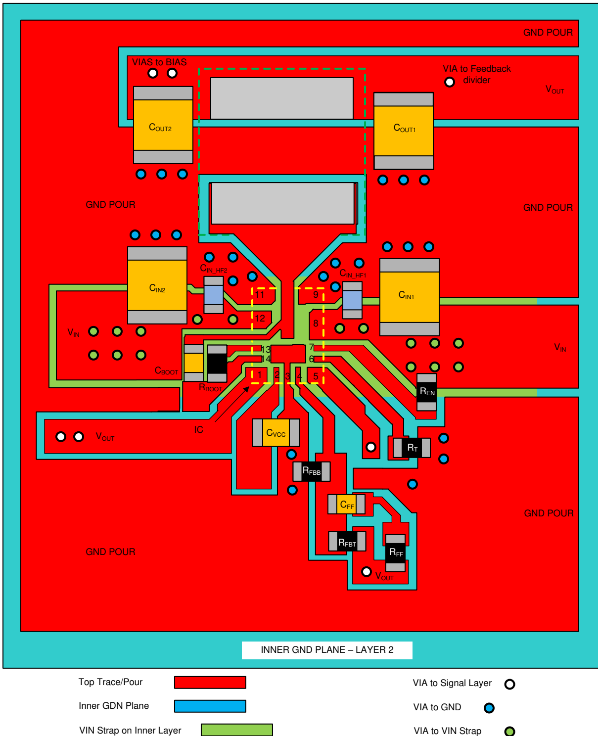
图 11-2. Layout Example
