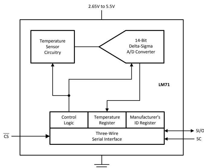
ブロック概略図
