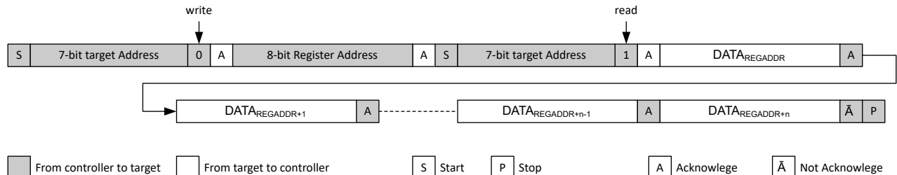
図 8-36. 定義されたレジスタ アドレスから開始されるシーケンシャル READ
