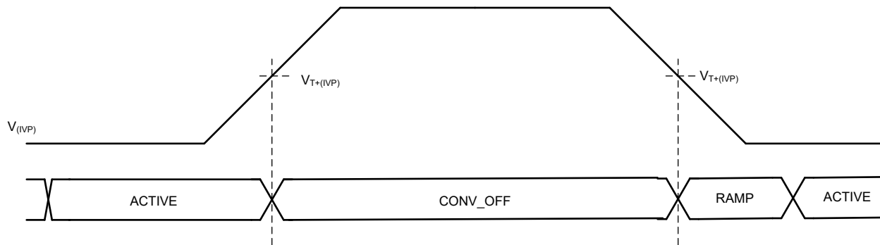
図 8-30. IVP 動作のタイミング図
