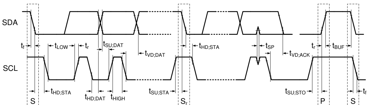
図 8-33. I 2 C データ送信タイミング
