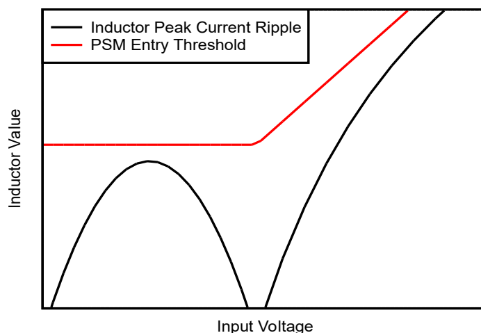
図 8-8. PSM エントリスレッショルドおよびリップル電流と入力電圧との関係を示す一般的なグラフ
