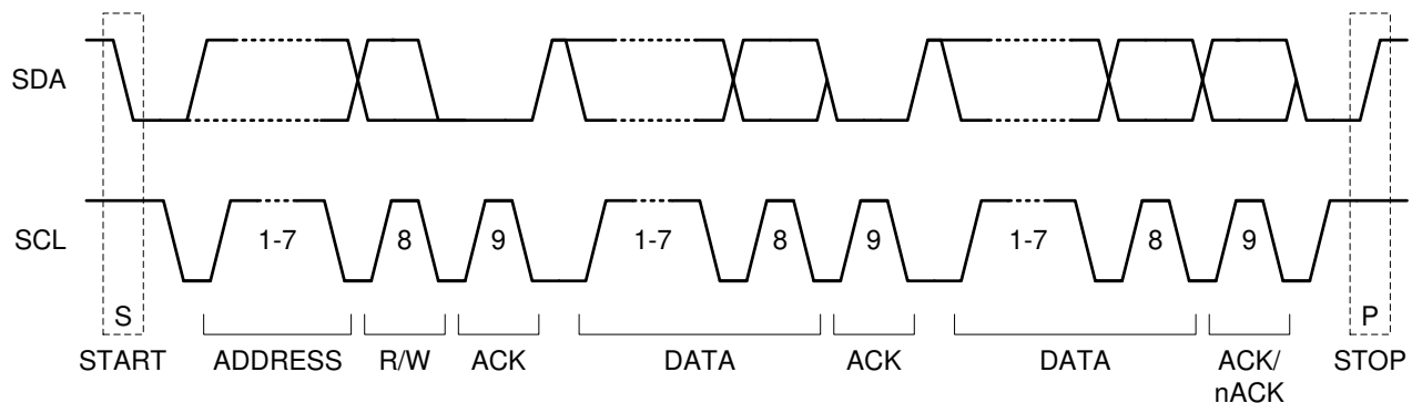
図 8-32. I 2 C スタート/ストップ/アクノリッジのプロトコル
