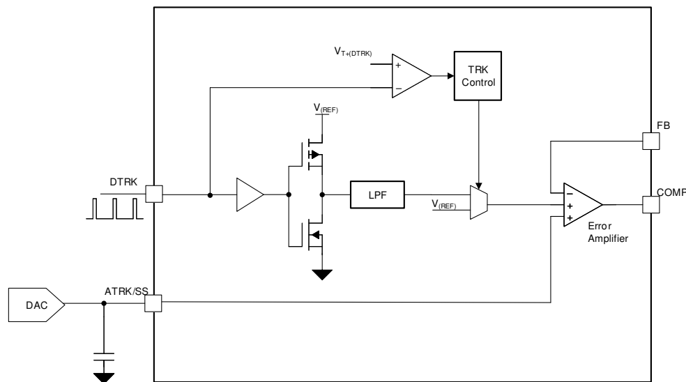
図 8-23. 出力電圧トラッキングの機能ブロック図
