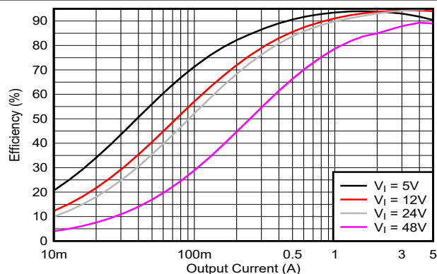
図 10-3. 効率と I_O との関係 (MODE = VCC2, V_O = 12V )
