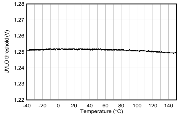
図 6-14. EN/UVLO スレッシュホールドと温度との関係
