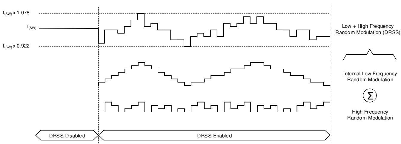
図 8-25. デュアル ランダム スペクトラム拡散
