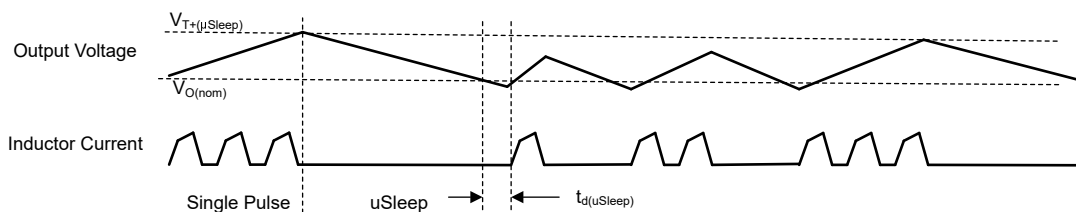
図 8-7. パワーセーブモード (μSleep 有効) のタイミング図
