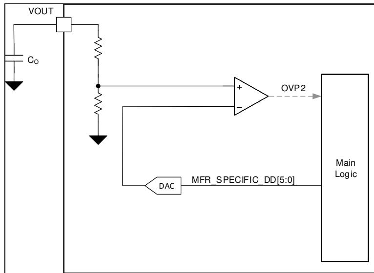
図 8-29. OVP2 の機能ブロック図
