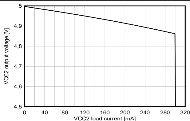
図 6-11. VCC2 LDO 出力電圧と VCC2 負荷電流との関係 V_{(VIN)} = 3.5\text{V} 、 V_{(BIAS)} = 12\text{V}
