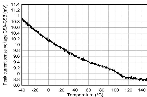
図 6-28. 平均電流制限スレッシュホールド電圧と温度との関係 ILIM_THRESHOLD = 0x14
