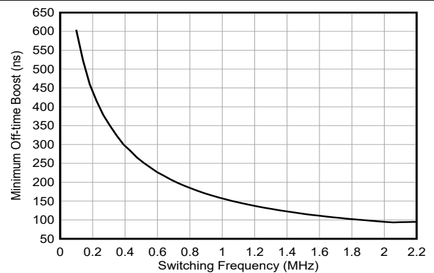
図 6-18. 昇圧の最小オフ時間とスイッチング周波数との関係
