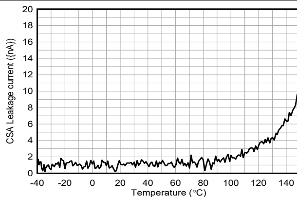
図 6-24. CSA 入力電流と温度との関係
