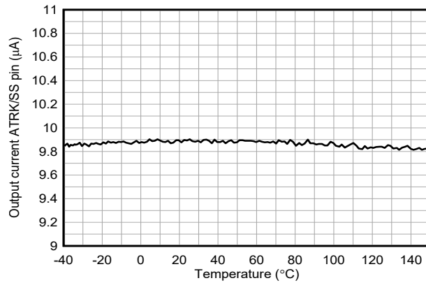
図 6-13. ソフト スタート電流と温度との関係
