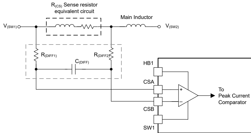
図 8-16. ピーク電流センサの概略回路図
