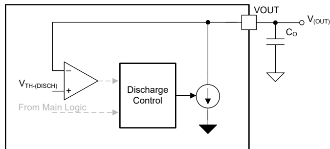
図 8-15. 機能ブロック図出力放電
