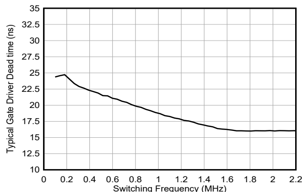
図 6-21. ゲートドライバ遅移 (デッド) 時間とスイッチング周波数との関係
