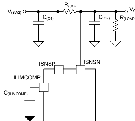
図 8-18. 抵抗性負荷を備えた電流制限部品の概略回路図
