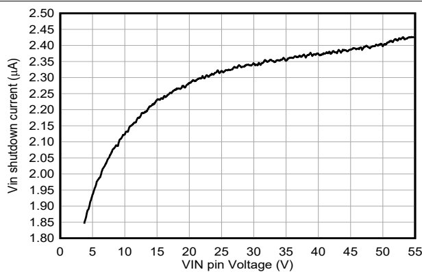
図 6-5. VIN へのシャットダウン電流とピン電圧との関係 V EN/UVLO = 0V、V (VIN) = 12V、V (BIAS) = 0V
