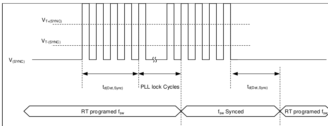
図 8-22. タイミング図の同期機能
