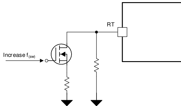
図 8-19. 周波数ホッピングの例
