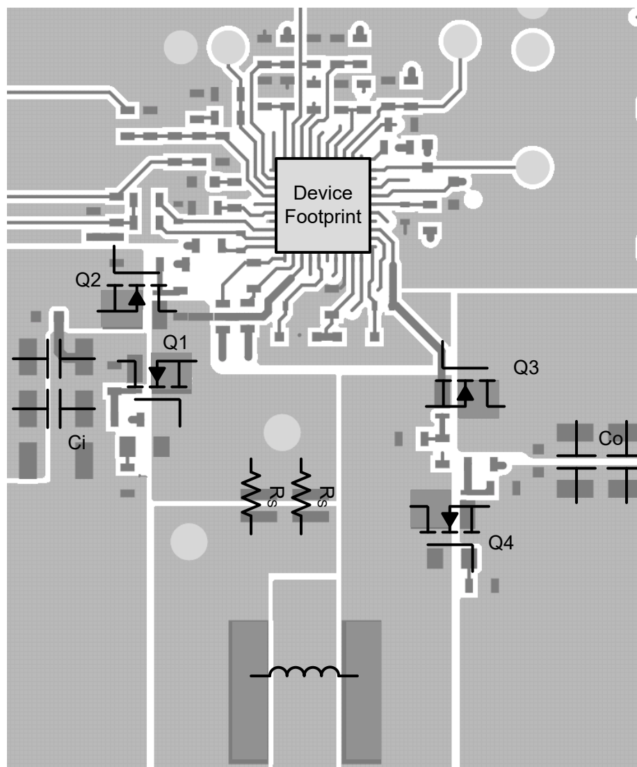
図 10-29. LM851772-Q1 の簡略上層の例
