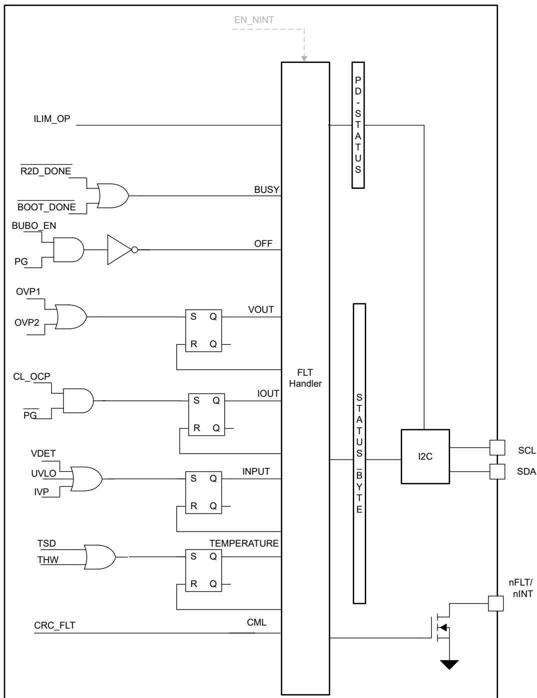
図 8-28. 機能ブロック図フォルト ハンドラ
