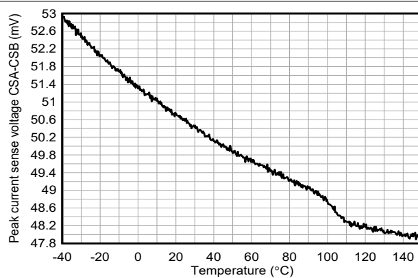
図 6-26. 平均電流制限スレッシュホールド電圧と温度との関係 ILIM_THRESHOLD = 0x64
