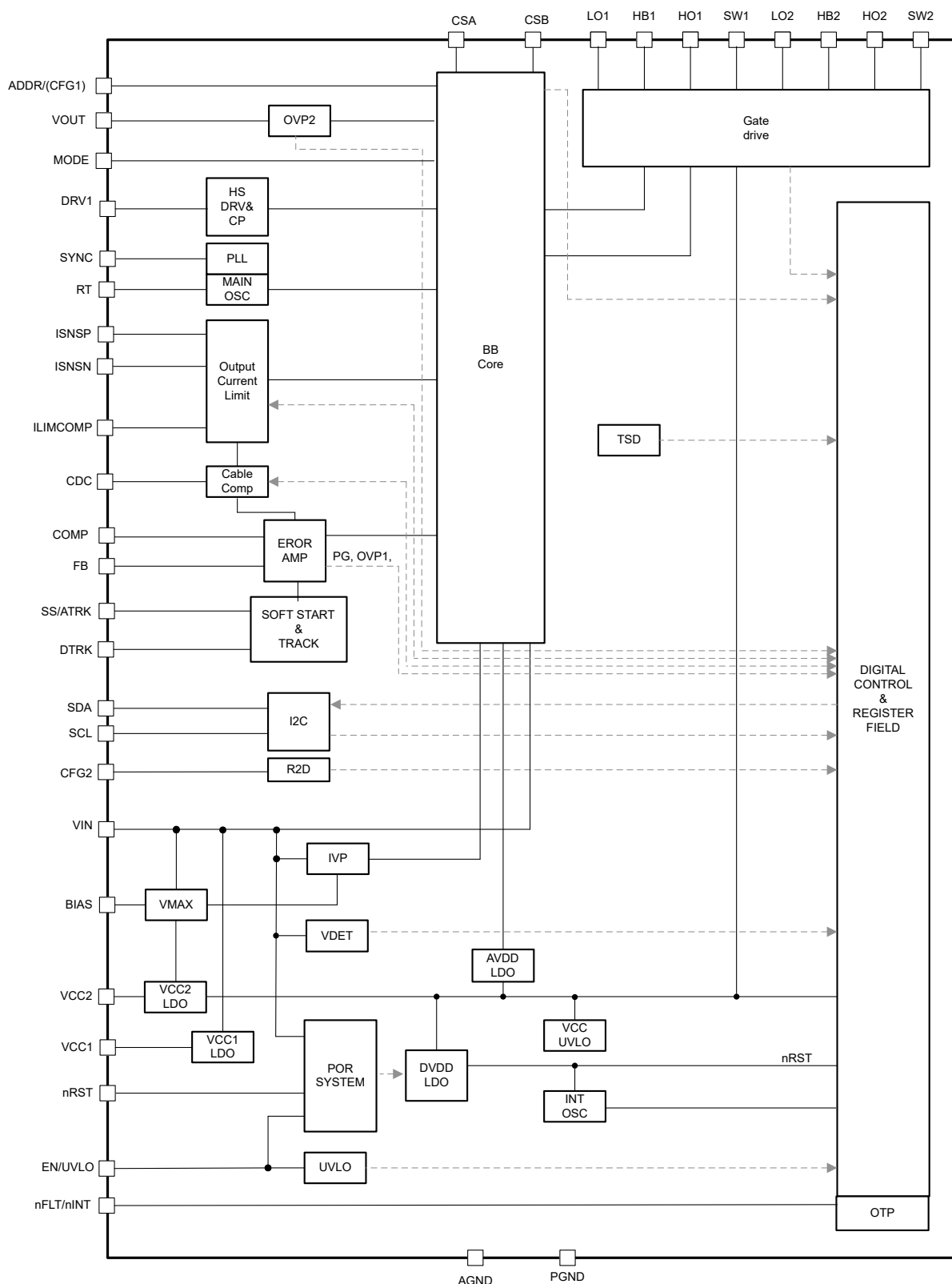
図 8-1. LM851772-Q1 機能ブロック図
