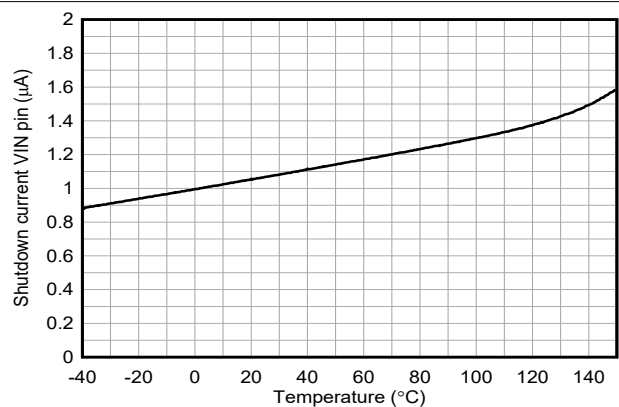
図 6-6. VIN へのシャットダウン電流と温度との関係 V EN/UVLO = 0V、V (VIN) = 12V、V (BIAS) = 0V
