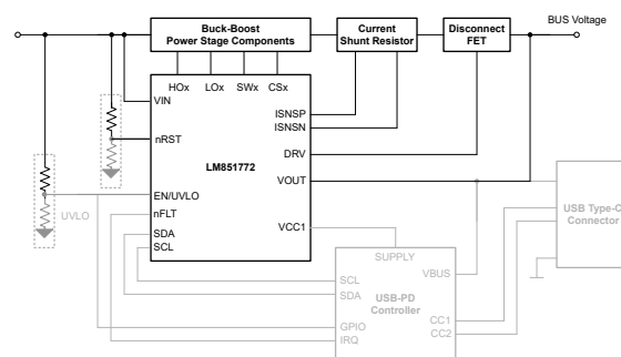
代表的なアプリケーション回路図
