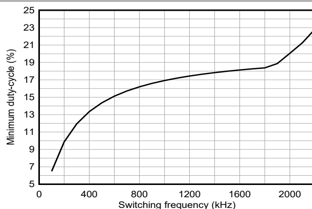
図 6-20. PSM 動作の降圧最小デューティ サイクルとスイッチング周波数との関係 (SYNC_OUT = イネーブル)
