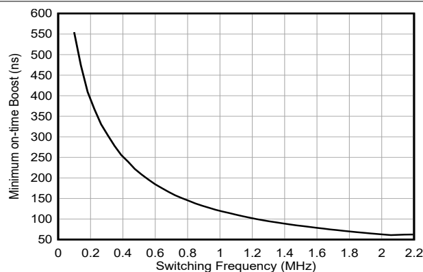
図 6-19. 昇圧の最小オン時間とスイッチング周波数との関係
