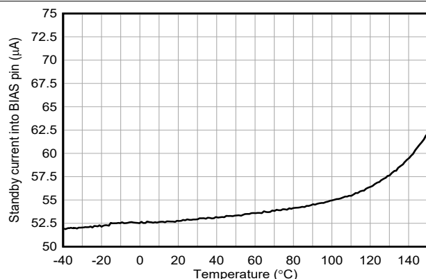
図 6-10. BIAS へのスタンバイ電流と温度との関係 V_{(VIN)} = 3.5\text{V} V_{(VIN)} = 12\text{V}
