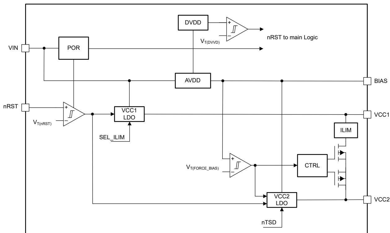
図 8-9. 機能ブロック図リファレンス システム
