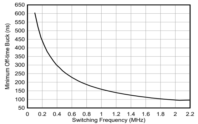
図 6-16. 降圧の最小オフ時間とスイッチング周波数との関係
