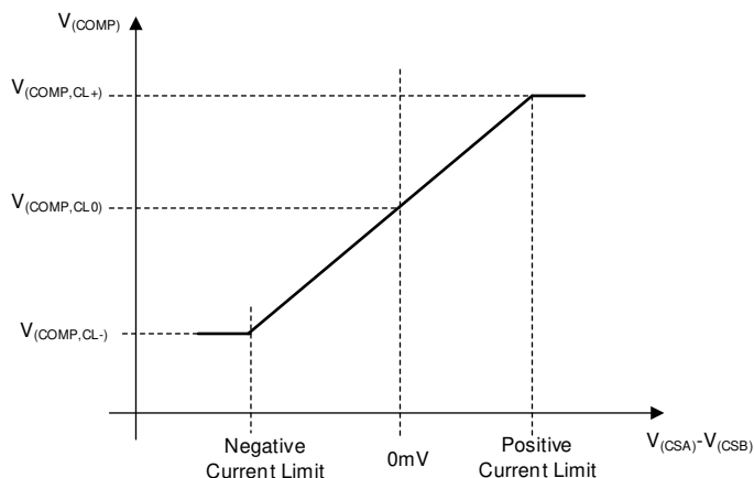
図 8-13. ピーク電流検出電圧と V_{COMP} との関係の制御機能
