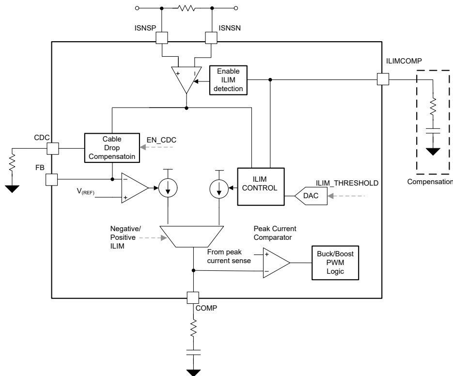
図 8-17. 電流モニタの機能ブロック図
