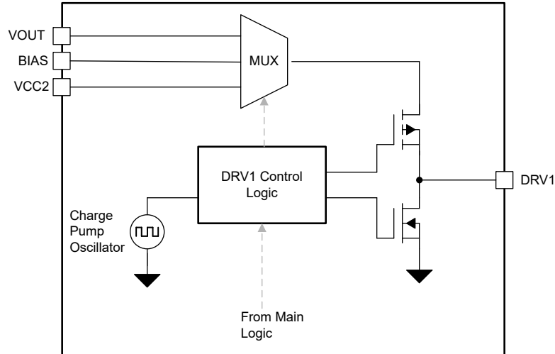
図 8-24. 機能ブロック図 - DRV ピン
