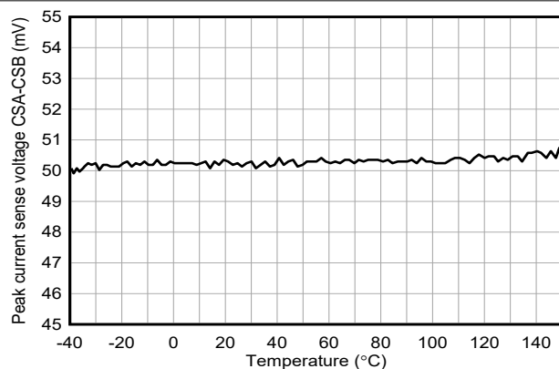
図 6-23. ピーク電流制限スレッシュホールド電圧と温度との関係
