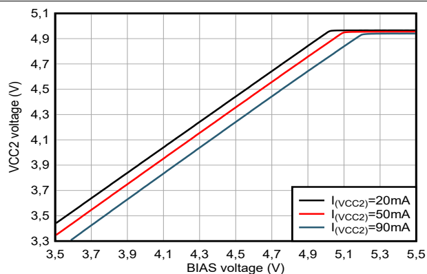
図 6-12. VCC2 LDO 出力電圧と BIAS 電圧との関係 V_{(VIN)} = 2.5\text{V}
