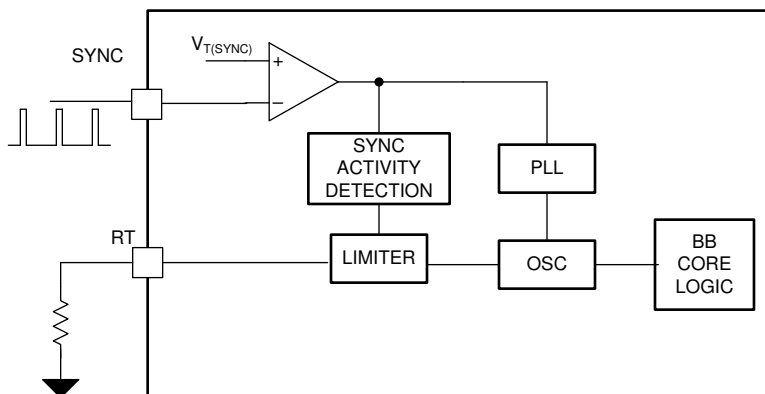
図 8-21. メイン発振器の機能ブロック図
