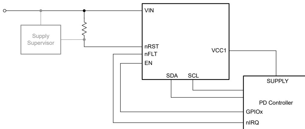
図 8-10. 概略回路図
