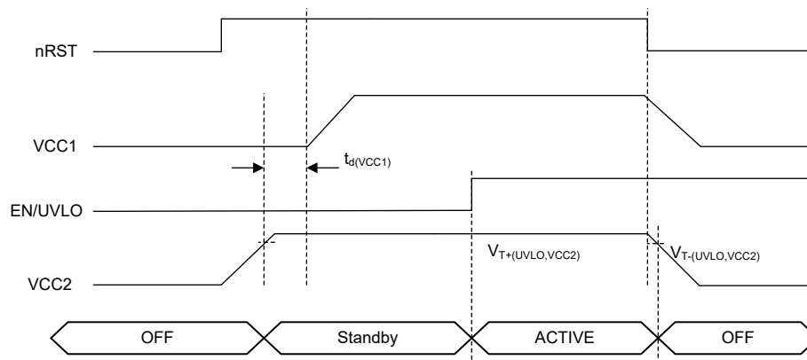
図 8-11. VCC レギュレータのタイミング図
