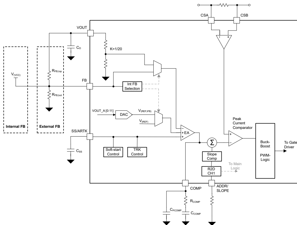
図 8-14. EA 機能ブロック図
