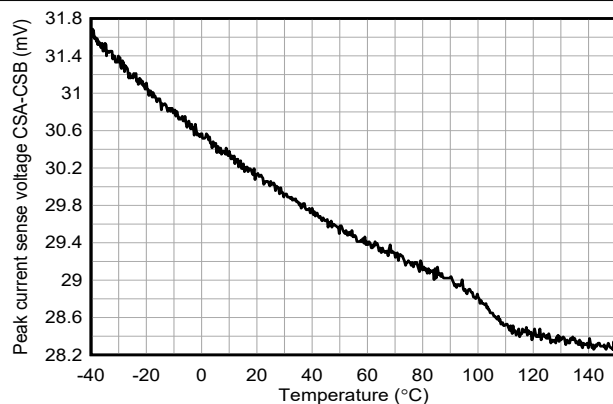
図 6-27. 平均電流制限スレッシュホールド電圧と温度との関係 ILIM_THRESHOLD = 0x3C
