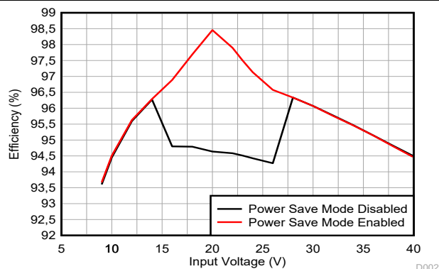
図 10-5. 効率と V_I ( V_O = 20V , I_O = 5A )
