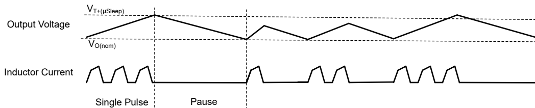
図 8-6. パワーセーブモード (μSleep 無効) のタイミング図
