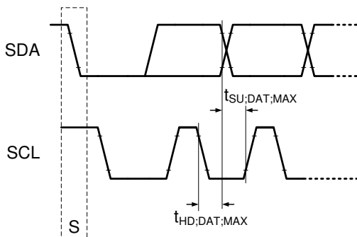
図 8-34. 最大の立ち上がり/立ち下がり時間の I 2 C データ送信タイミング
