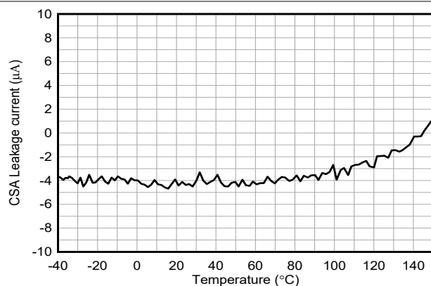
図 6-25. CSB 入力電流と温度との関係
