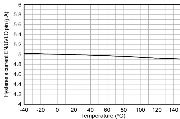
図 6-15. EN/UVLO のヒステリシス電流と温度との関係
