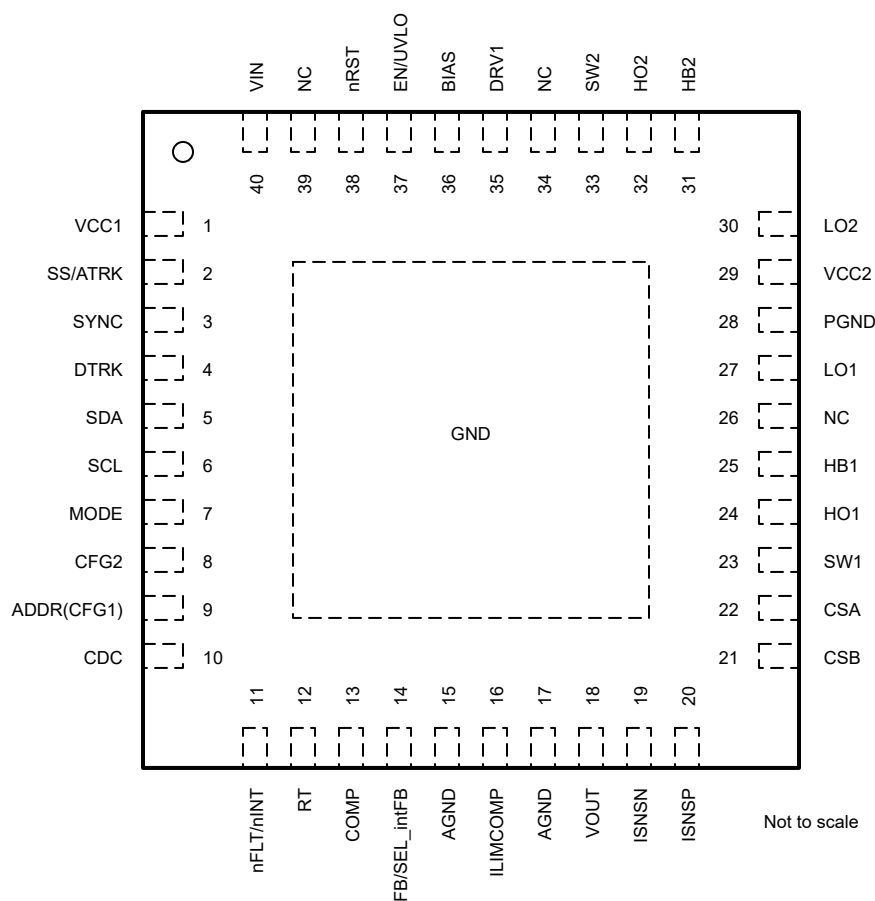
図 5-1. LM851772-Q1 RHA パッケージ、40 ピン QFN (上面図)
