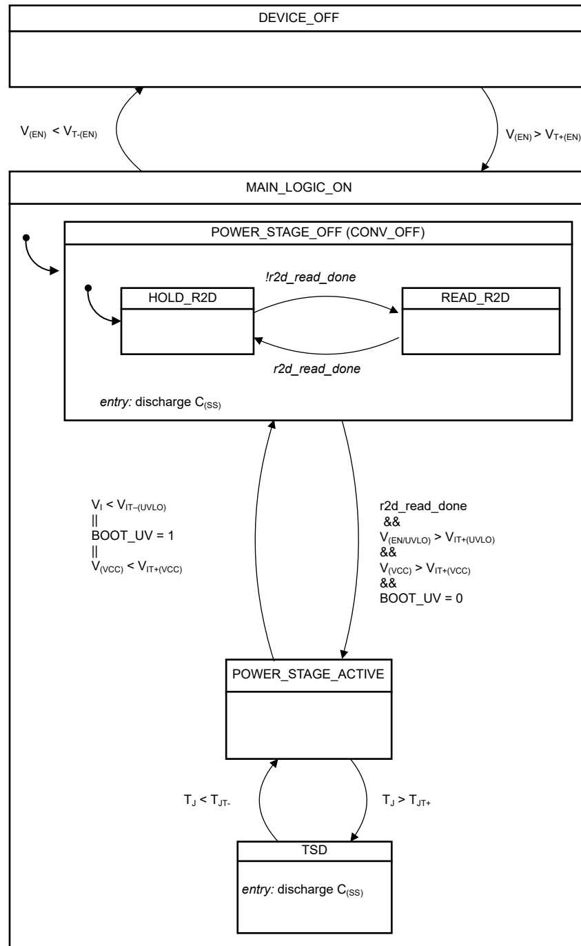
図 8-31. 状態遷移図
