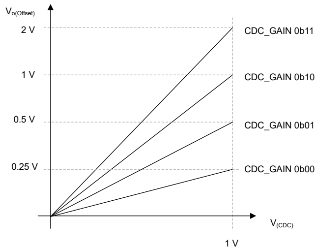
図 8-27. Vo オフセットと CDC 電圧との関係
