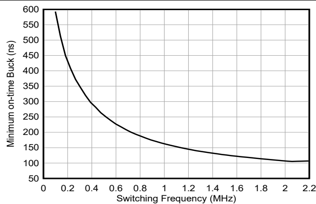
図 6-17. 降圧の最小オン時間とスイッチング周波数との関係
