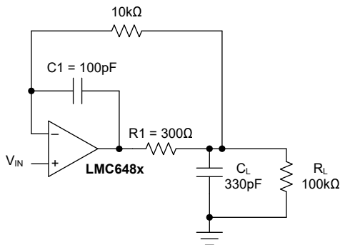
図 7-6. 300pF の容量性負荷および 100kΩ の抵抗性負荷に対応するよう補償された非反転型アンプ
