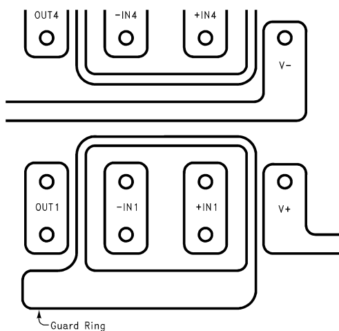
図 7-20. PC のガード リングの例基板レイアウト
