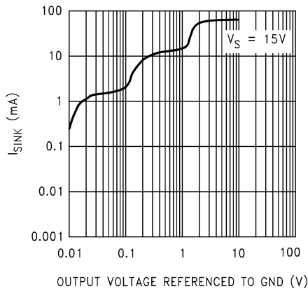
図 6-7. シンク電流と出力電圧との関係
