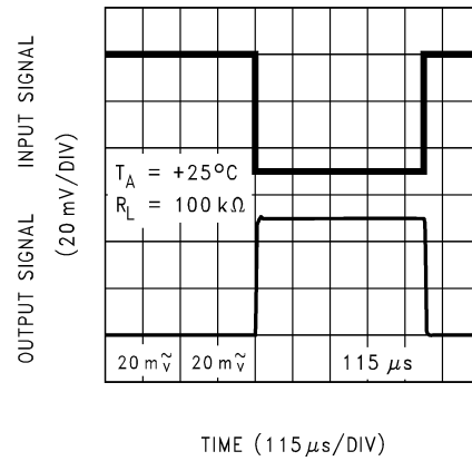
図 6-26. 反転型の小信号パルス応答
