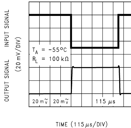
図 6-27. 反転型の小信号パルス応答
