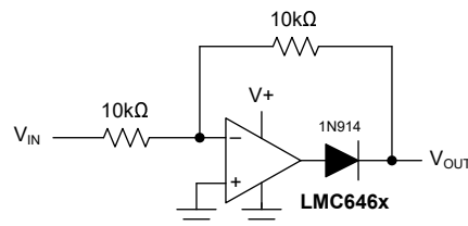
図 7-16. 全波整流器、入力電流保護 (R i ) 付き
