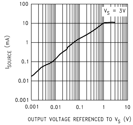
図 6-2. ソース電流と出力電圧との関係
