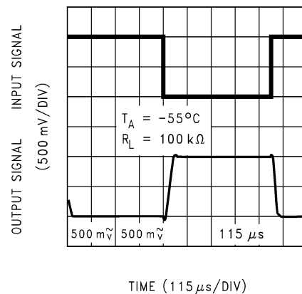
図 6-24. 反転型の大信号パルス応答
