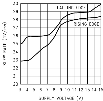
図 6-15. スルーレートと電源電圧との関係
