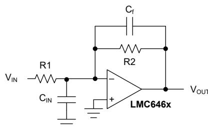
図 7-8. 入力容量の影響の相殺
