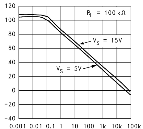
図 6-12. 開ループの周波数応答
