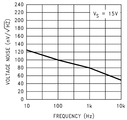
図 6-8. 入力電圧ノイズと周波数との関係
