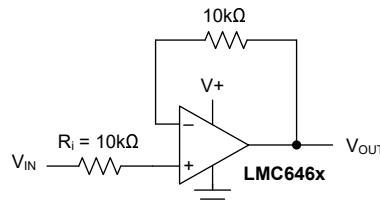
図 7-15. 半波整流器、入力電流保護 (R i ) 付き
