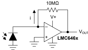
図 7-13. 光検出回路
