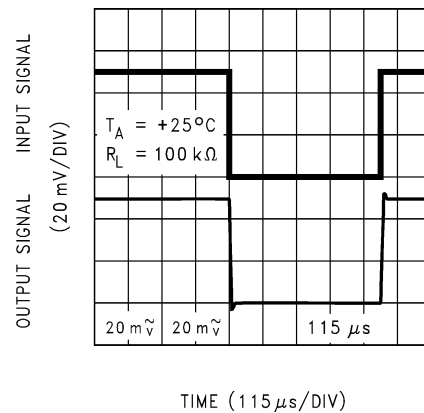
図 6-20. 非反転型の小信号パルス応答
