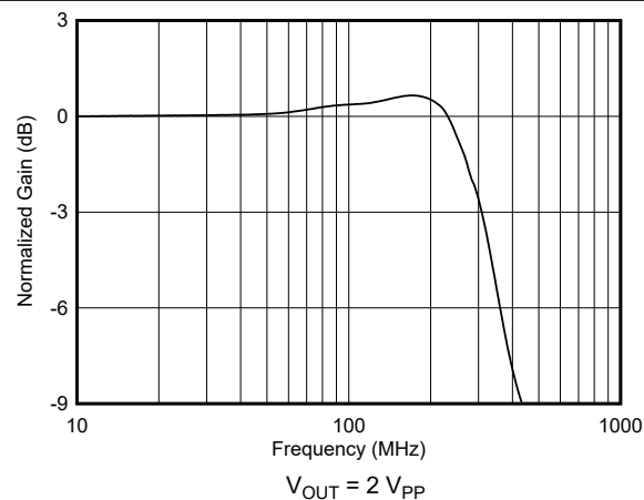
図 6-2. 大信号周波数応答
