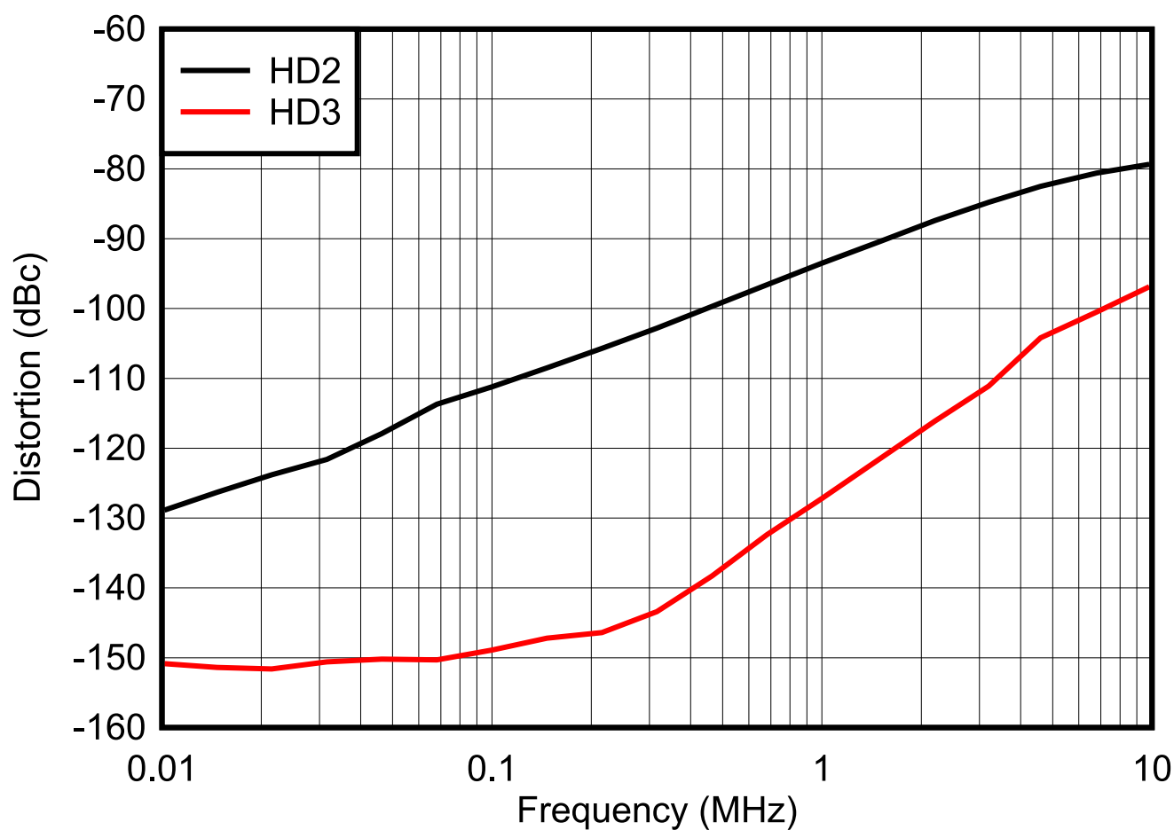
高調波歪みと周波数との関係
