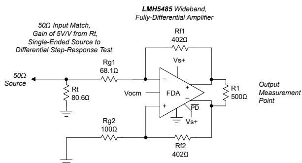
図 7-2. DC 結合、シングルエンドから差動、ゲイン 5V/V に設定した基本的なテスト回路
