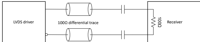
図 7-8. AC 終端 LVDS 出力
