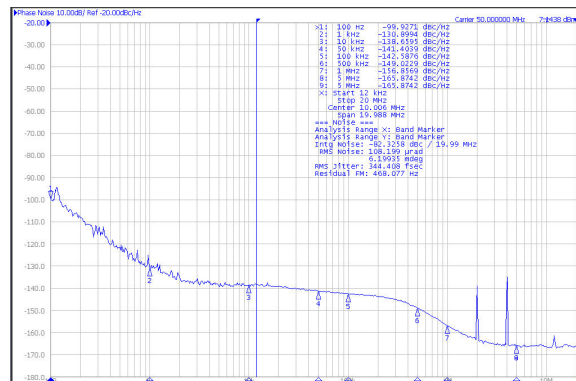
図 6-20. 50MHz HSDS Output From APLL1
