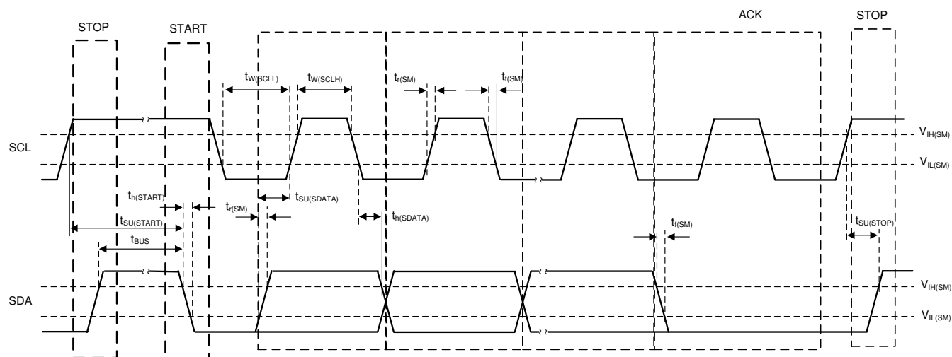
图 6-4. I 2 C Timing Diagram
