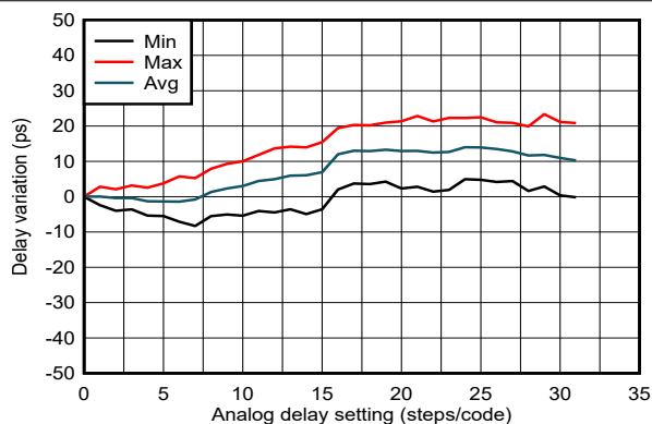
図 6-23. SYSREF/1PPS Delay Linearity vs. Analog Delay Code 4
