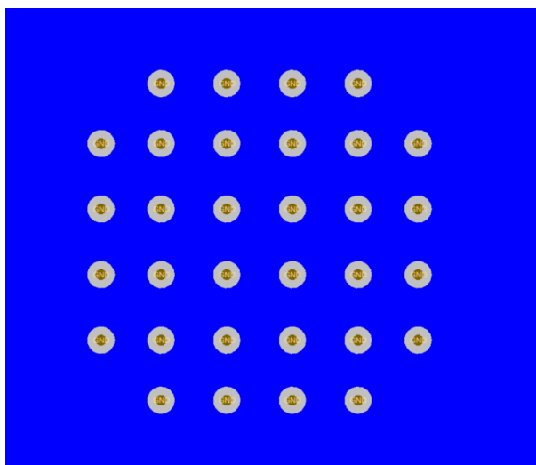
図 9-6. PCB Layout Example for LMK5C33216AS1, Bottom Layer
