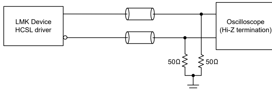
図 7-7. HCSL Output Time Domain Test Configuration
