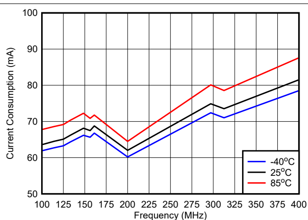
図 6-8. 消費電流と周波数との関係 (HCSL、3.3V)
