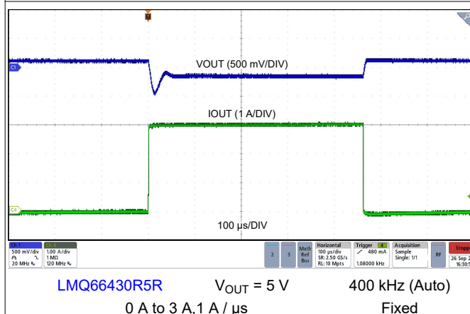
9-8. Load Transient
