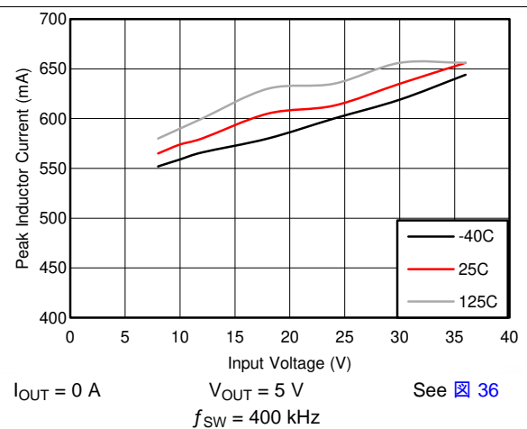
图 6. I_{PEAK-MIN}
