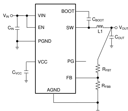
概略回路図
