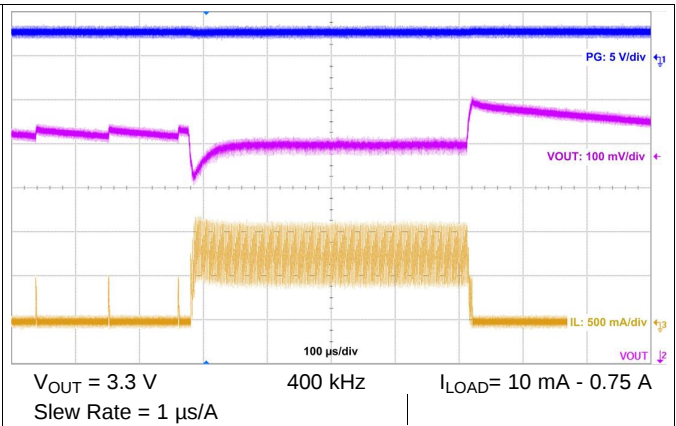
図 35. Load Transient
