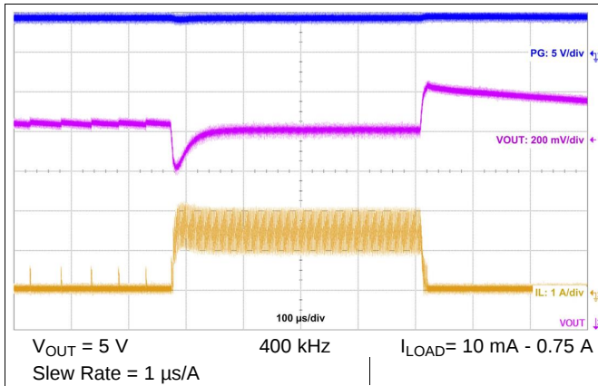
図 34. Load Transient
