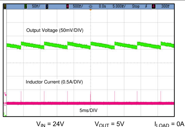
図 8-20. 無負荷時での出力リップル
