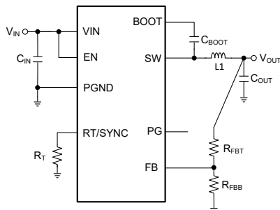
概略回路図
