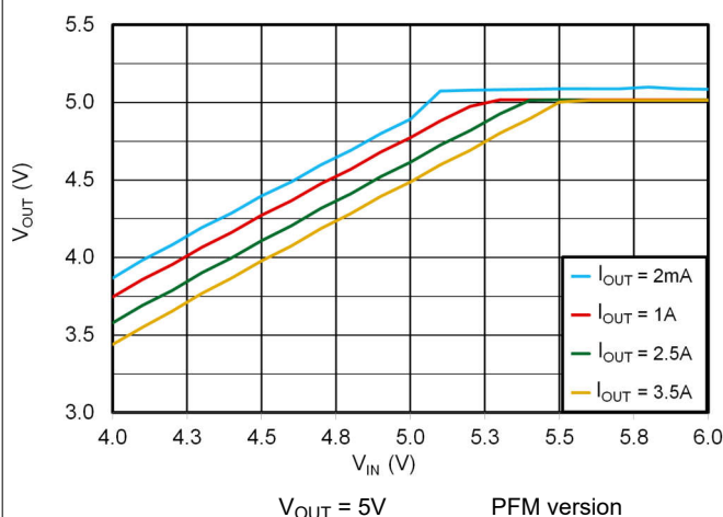
図 6-11. 5V Dropout
