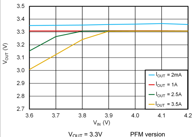
図 6-12. 3.3V Dropout
