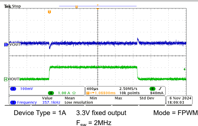
8-7. 0A to 1A Load Transient
