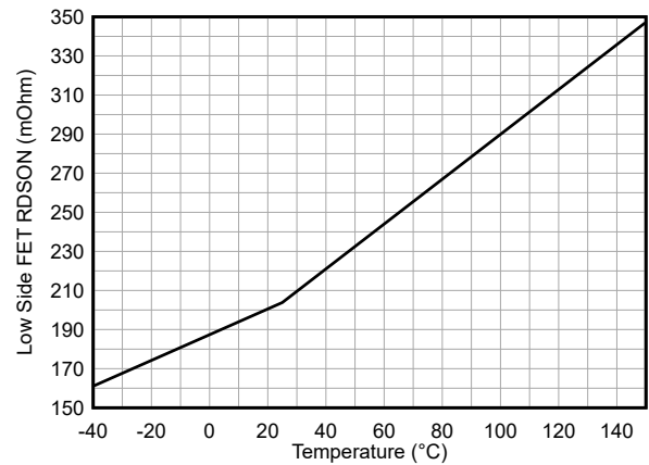
図 6-4. Low Side MOSFET RDSON vs Temperature
