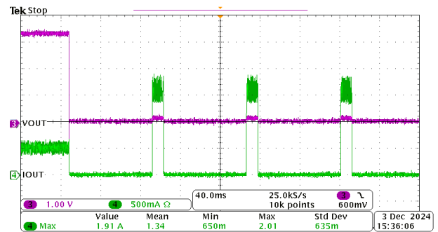
図 8-9. Short-Circuit Applied
