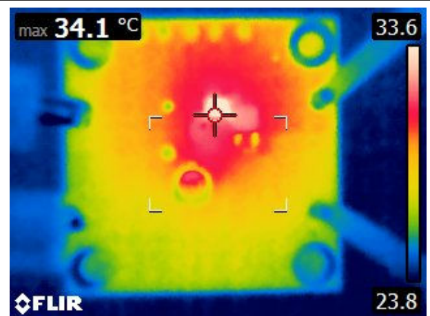
図 8-9. Short-Circuit Applied
