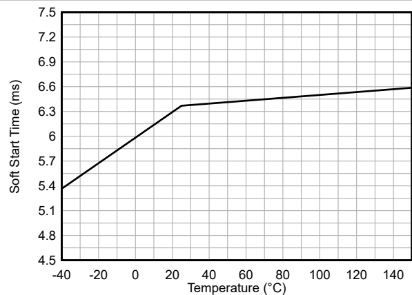
図 6-6. Soft Start Time vs Temperature
