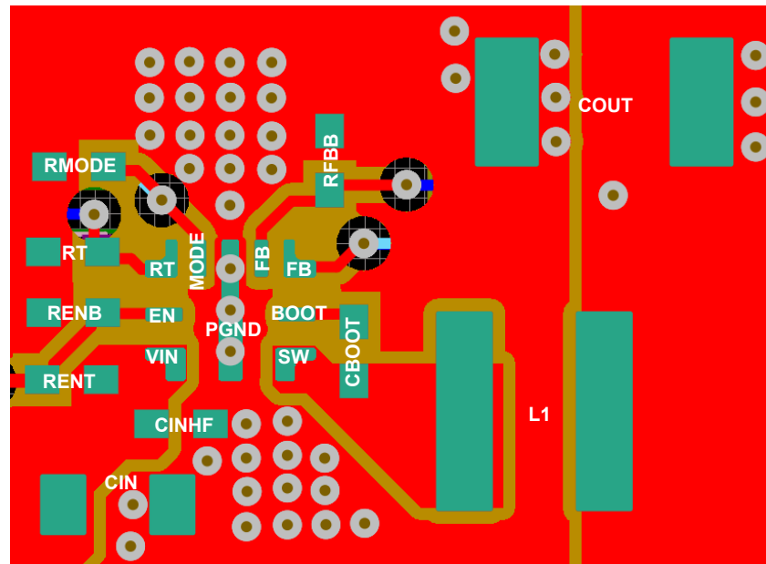
図 8-13. Example Layout
