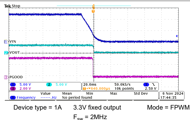
8-6. Shutdown
