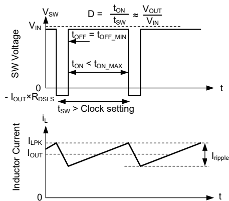
図 7-11. ドロップアウト波形
