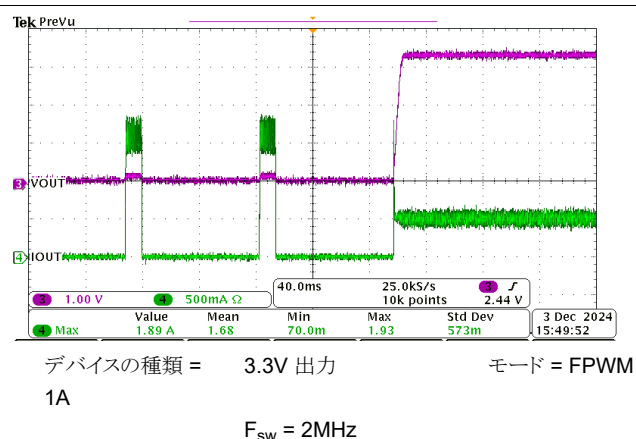
図 8-23. 短絡からの回復
