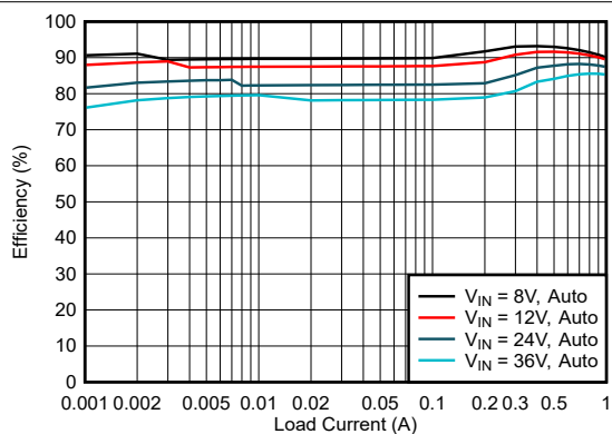
図 8-6. 効率
