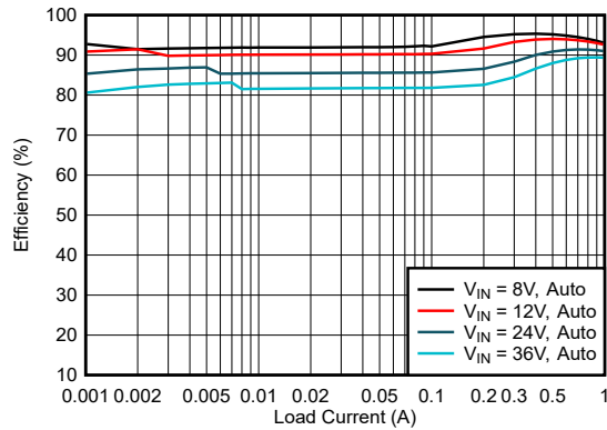
図 8-2. 効率
