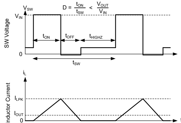
図 7-8. PFM 動作
