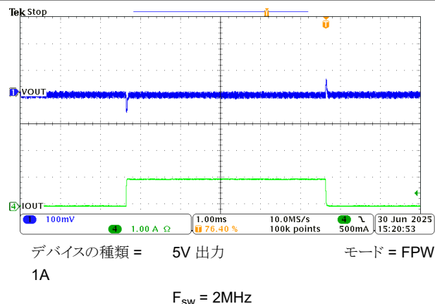
図 8-18. 0A ~ 1A の負荷過渡
