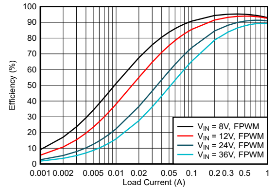
図 8-3. 効率
