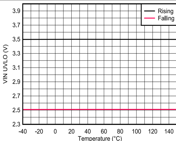
図 6-11. 入力電圧 UVLO - B バリエーション
