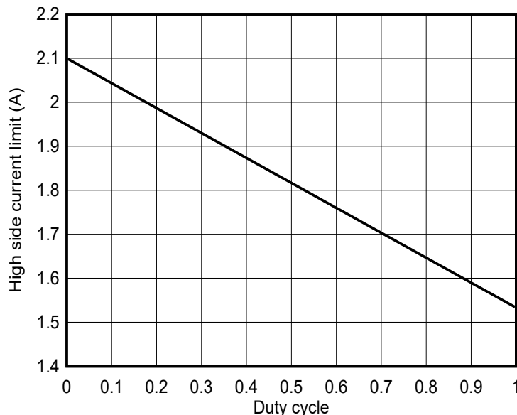
図 7-5. デューティ サイクル D の関数としての典型的なハイ サイド電流制限 I_{HS-LIM}
