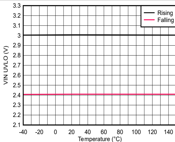
図 6-10. 入力電圧 UVLO - A バリエーション
