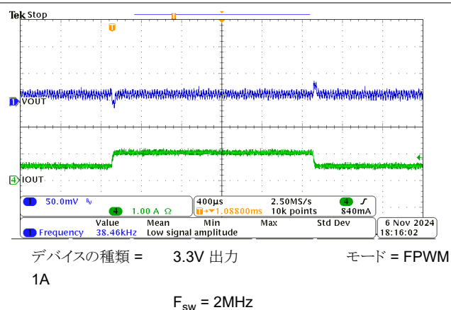
図 8-21. 0.5A ~ 1A の負荷過渡
