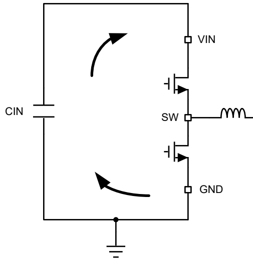
図 8-35. 高速過渡を持つ電流ループ
