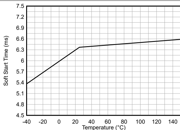
図 6-7. ソフト スタート時間
