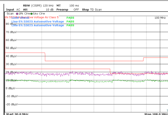
図 8-25. 伝導 EMI と CISPR25 制限値との関係 (紫: ピーク信号、緑: 平均信号)、LMR60410QEVM
