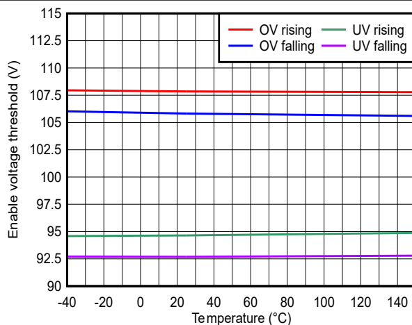
図 6-12. PGOOD スレッシュホールド
