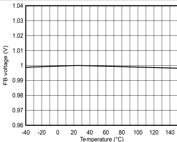
図 6-9. 帰還電圧精度
