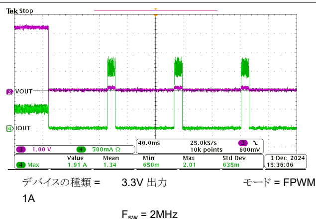
図 8-22. 短絡発生
