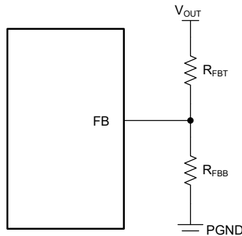
図 7-4. 可変 VOUT 用の帰還抵抗セットアップ
