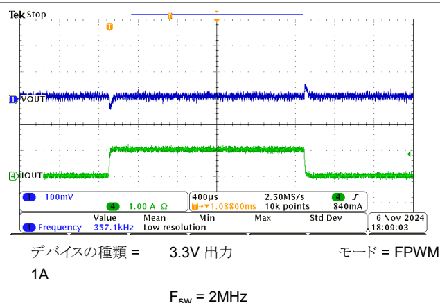
図 8-20. 0A ~ 1A の負荷過渡
