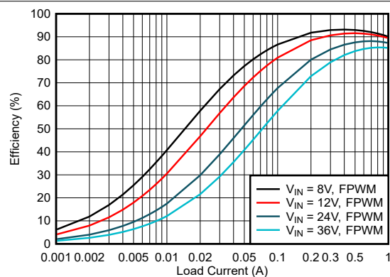
図 8-7. 効率
