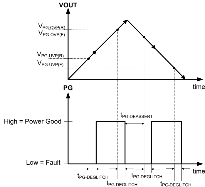
図 7-6. パワー グッド スレッシュホールド
