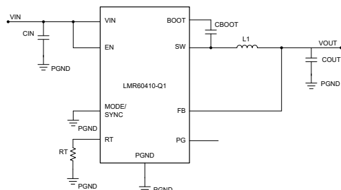
概略回路図 - 固定出力
