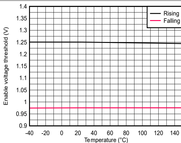
図 6-8. イネーブル スレッシュホールド電圧
