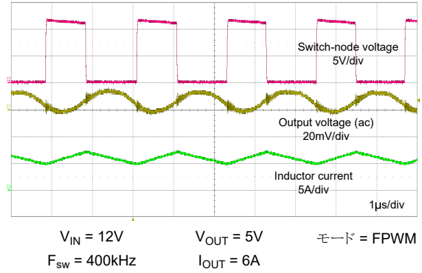
図 8-29. 定常状態のスイッチング波形と出力電圧リップル
