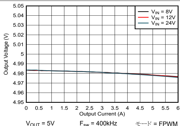
図 8-13. 負荷およびラインレギュレーション- FPWM モード
