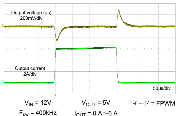
図 8-25. 負荷過渡
