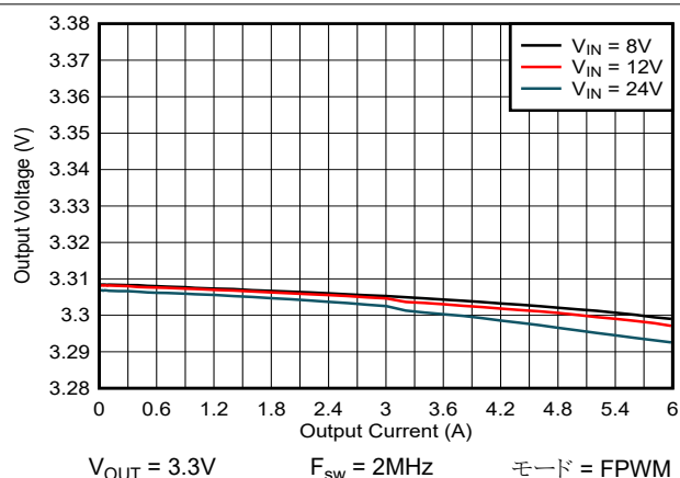
図 8-15. 負荷およびラインレギュレーション- FPWM モード
