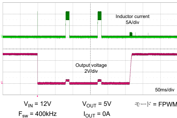
図 8-32. 短絡動作
