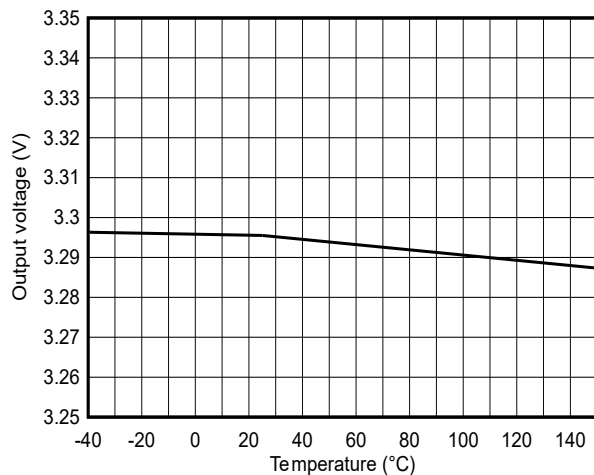
図 6-5. 出力電圧精度
