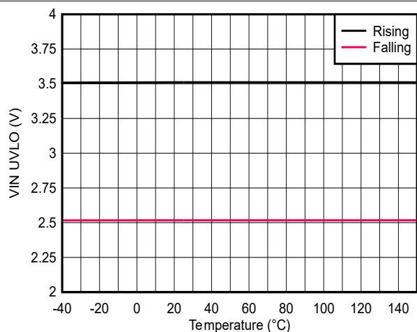
図 6-9. 入力電圧 UVLO
