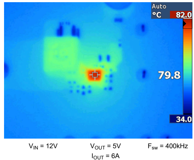
図 8-43. EVM の放熱特性
