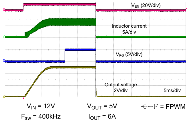
図 8-31. 6A 負荷でのスタートアップとシャットダウンの有効化
