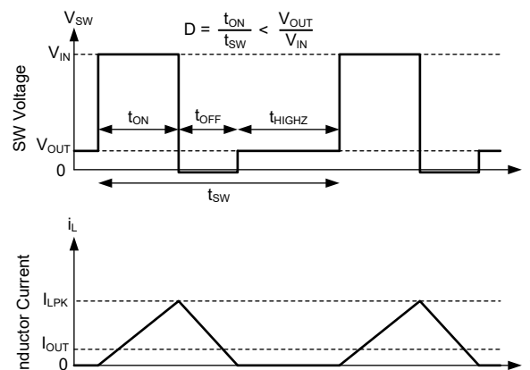
図 7-7. PFM 動作
