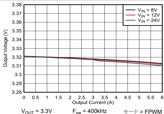
図 8-11. 負荷およびラインレギュレーション- FPWM モード
