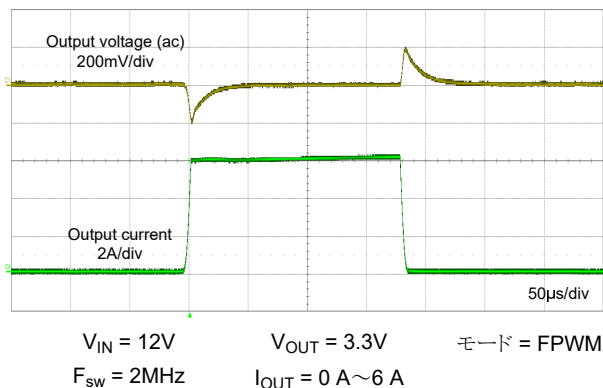
図 8-26. 負荷過渡
