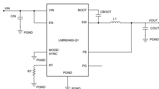
概略回路図 - 固定出力
