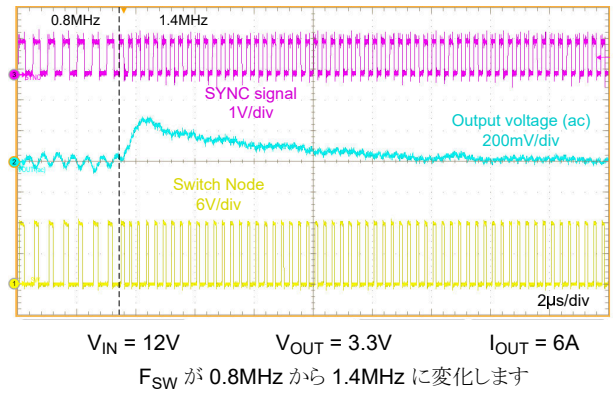
図 8-33. SYNC 周波数の過渡応答
