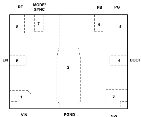
図 5-1. VBC パッケージ、9 ピン WQFN-FCRLF (上面図)
