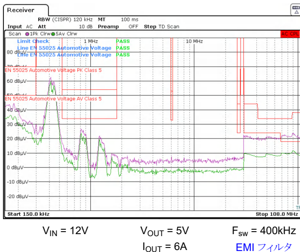
図 8-36. 伝導 EMI と CISPR 25 制限値との関係 (ピンク: ピーク信号、緑: 平均信号)
