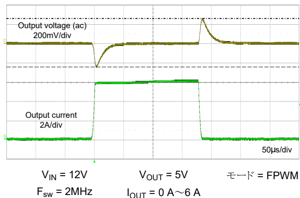
図 8-27. 負荷過渡
