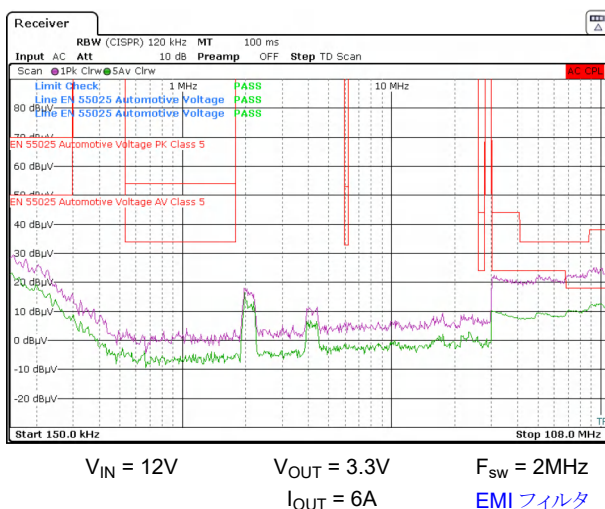
図 8-35. 伝導 EMI と CISPR 25 制限値との関係 (ピンク: ピーク信号、緑: 平均信号)
