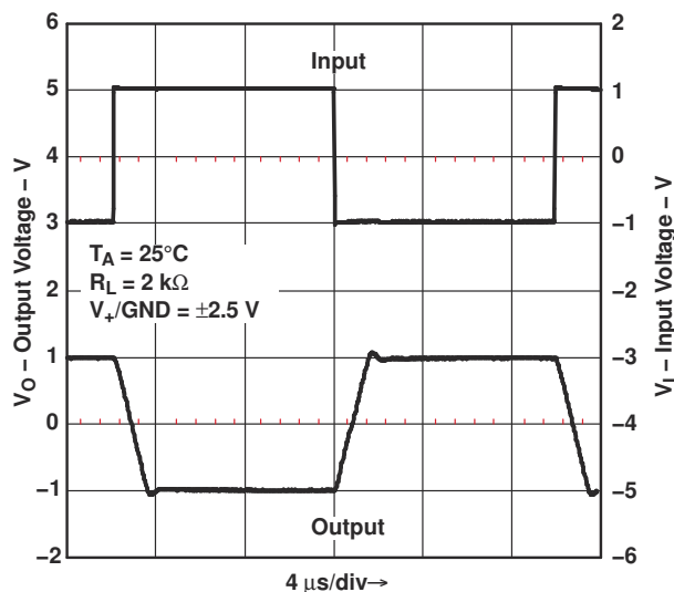
図 6-34. 大信号反転型応答
