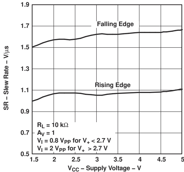
図 6-13. スルーレートと 電源電圧との 関係
