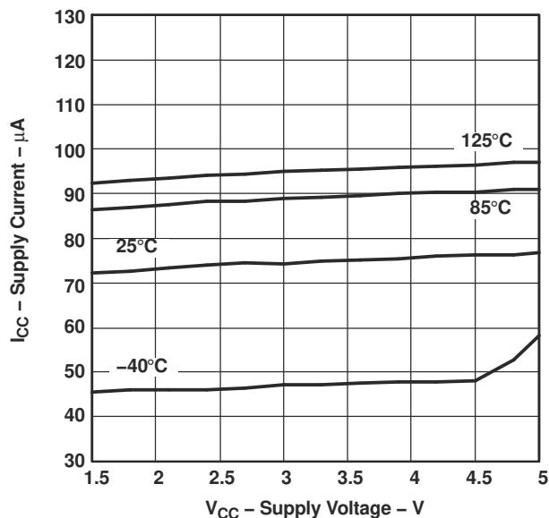
図 6-1. 電源電流と 電源電圧との 関係
