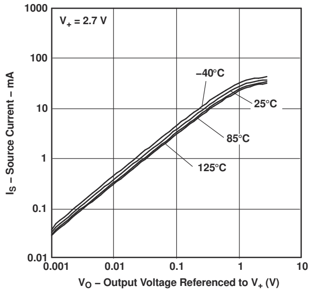
図 6-5. ソース電流と 出力電圧との 関係
