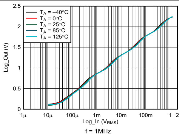
図 5-3. 各種温度ポイントとしての出力
