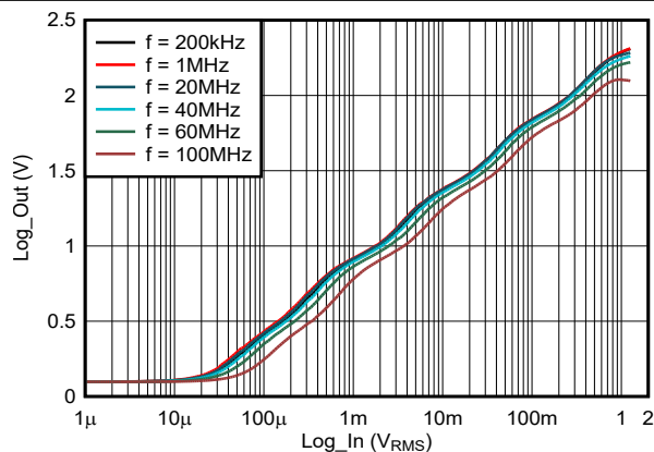
図 5-1. さまざまな周波数における出力
