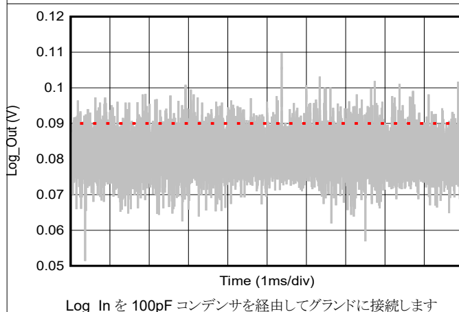
図 5-15. 最小 Log_Out 電圧と時間との関係
