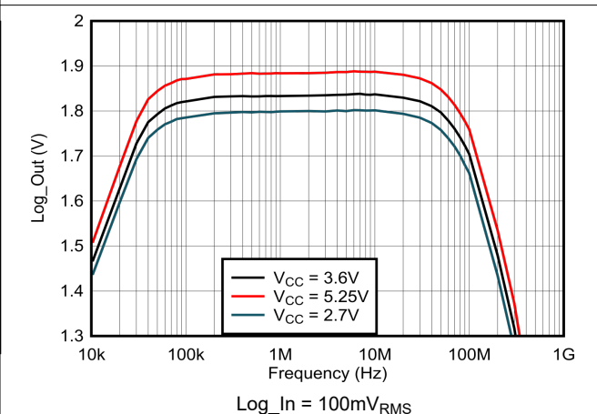
図 5-16. 出力変動
