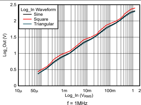
図 5-5. さまざまな入力波形に対する出力応答
