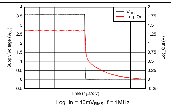
図 5-18. 電源ランプダウンのターンオフ時間
