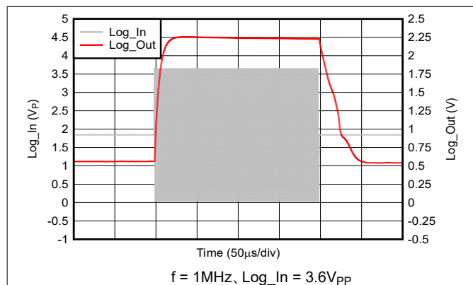
図 5-13. オーバードライブ復帰時間
