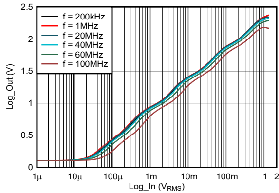
図 5-21. さまざまな周波数における出力
