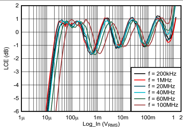
図 5-2. さまざまな周波数における対数適合誤差
