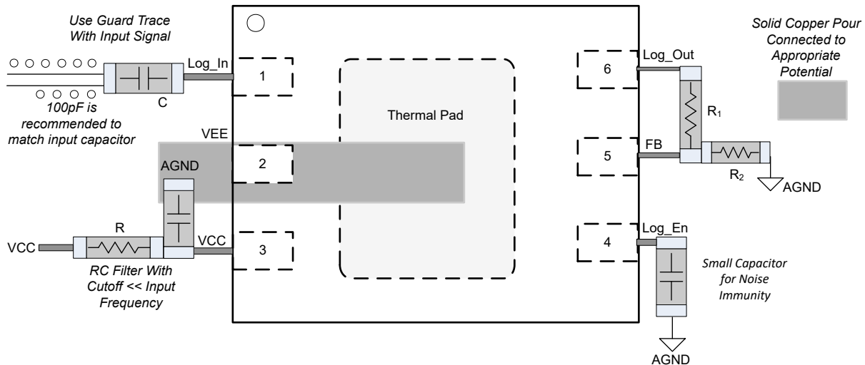
図 8-4. レイアウト例
