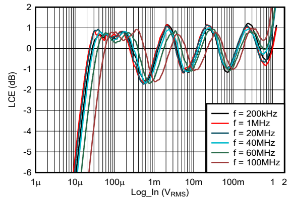
図 5-22. さまざまな周波数における対数適合誤差
