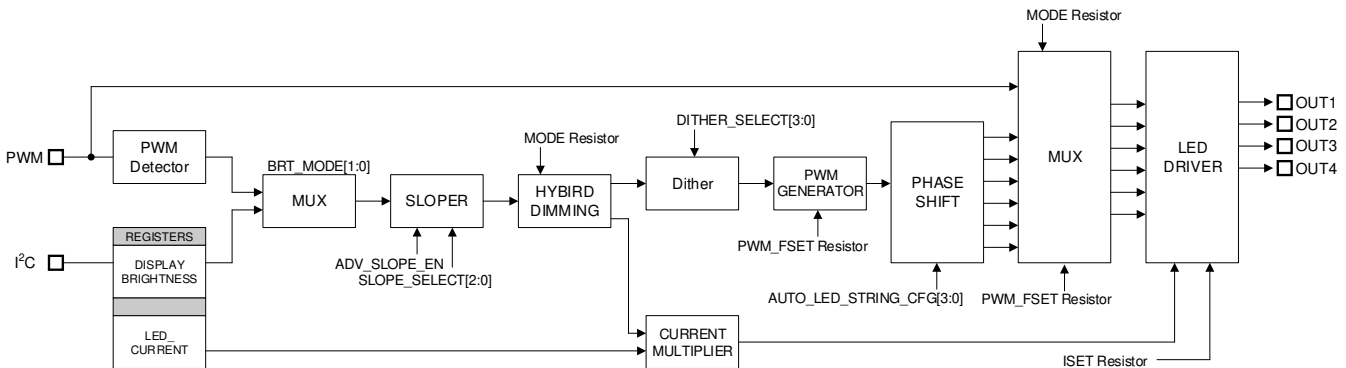
図 7-9. LP8864-Q1 Brightness Path Diagram
