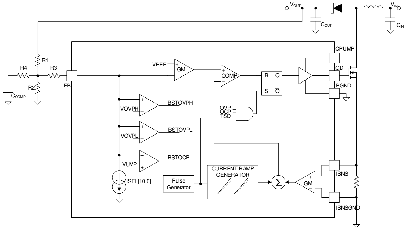
图 7-7. 外部补偿网络
