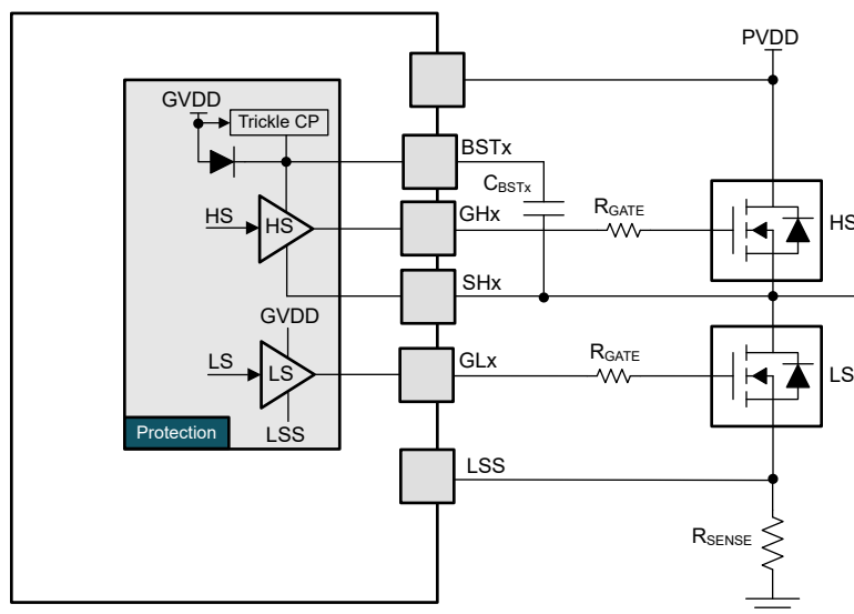
図 10-2. ゲート ドライバ出力 (直列抵抗を使用)
