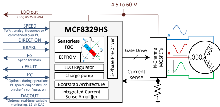
概略回路図
