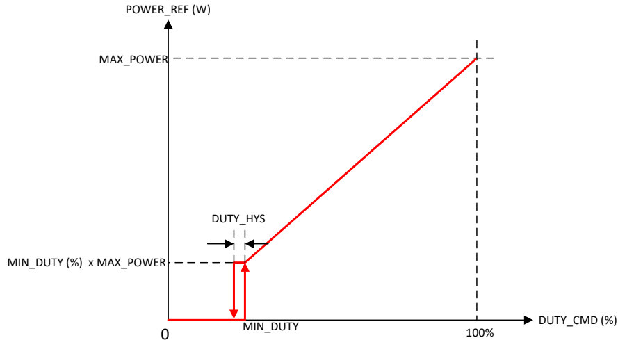
図 7-17. 電力リファレンスの伝達関数
