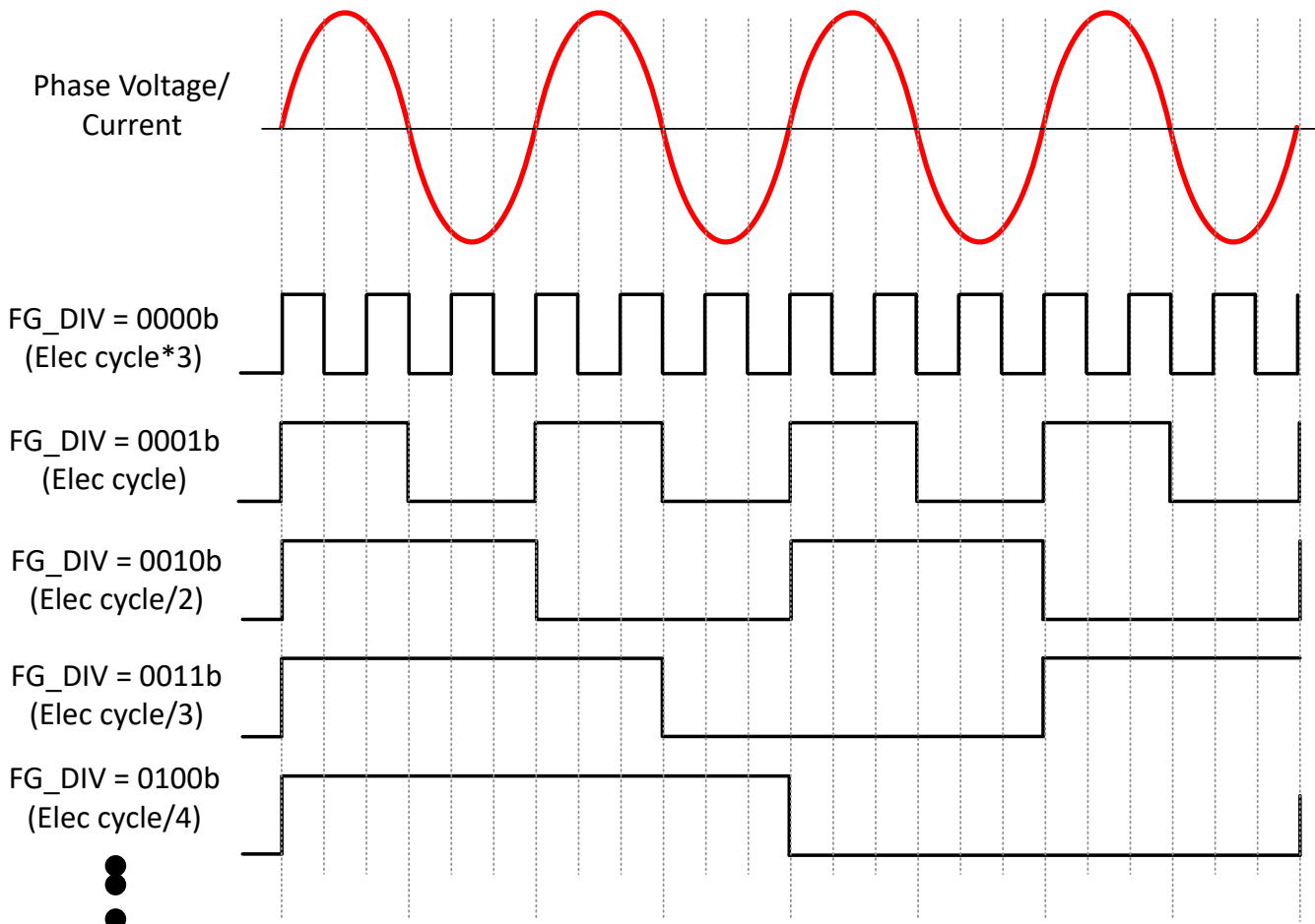
図 7-46. FG 分周器
