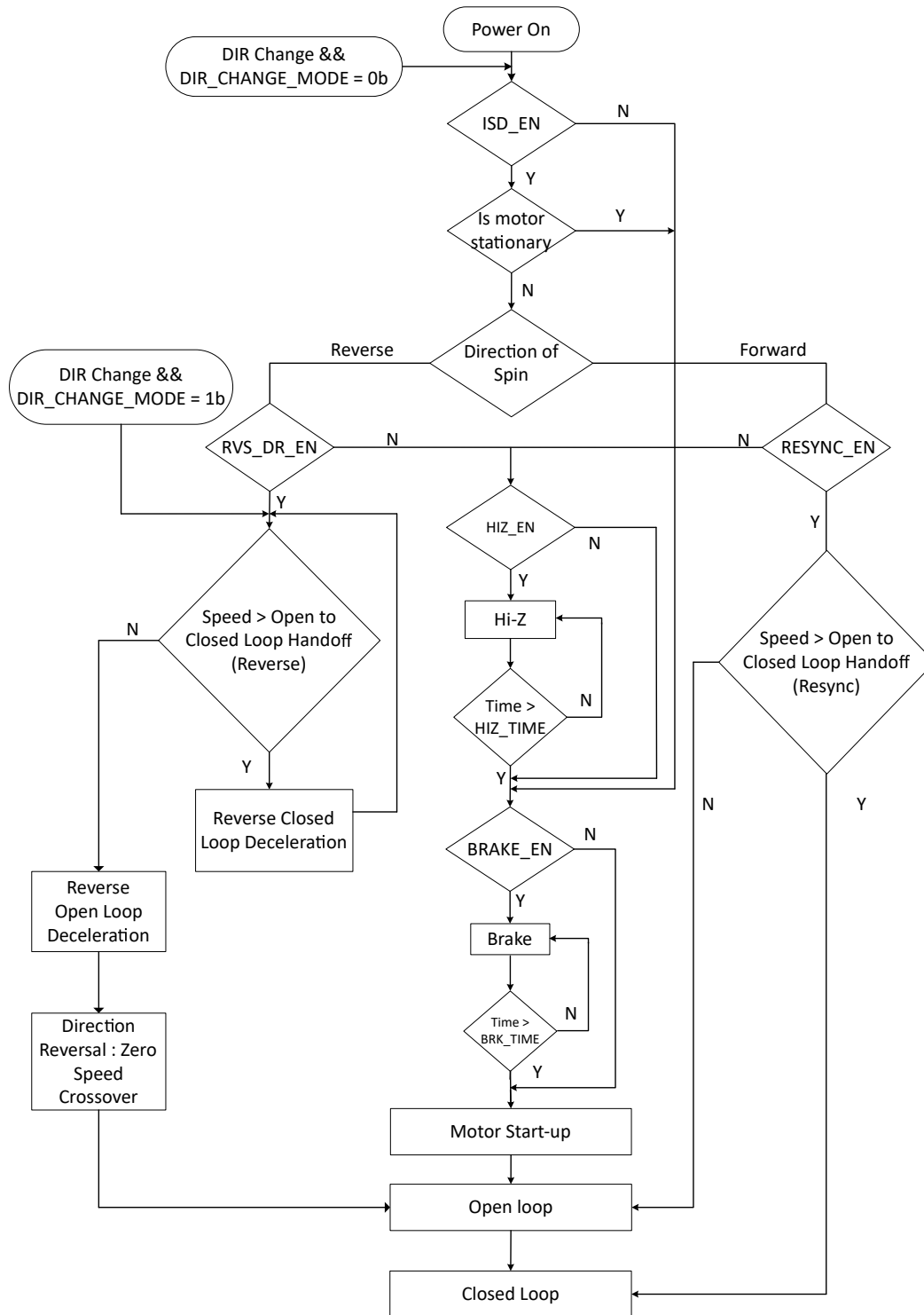
図 7-22. モーター起動フロー
