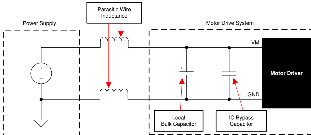
図 10-6. 外部電源を使用したモーター駆動システムの構成例
