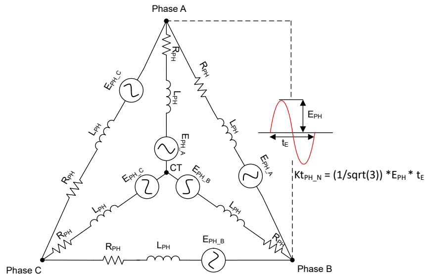
図 7-40. モーター逆起電力定数
