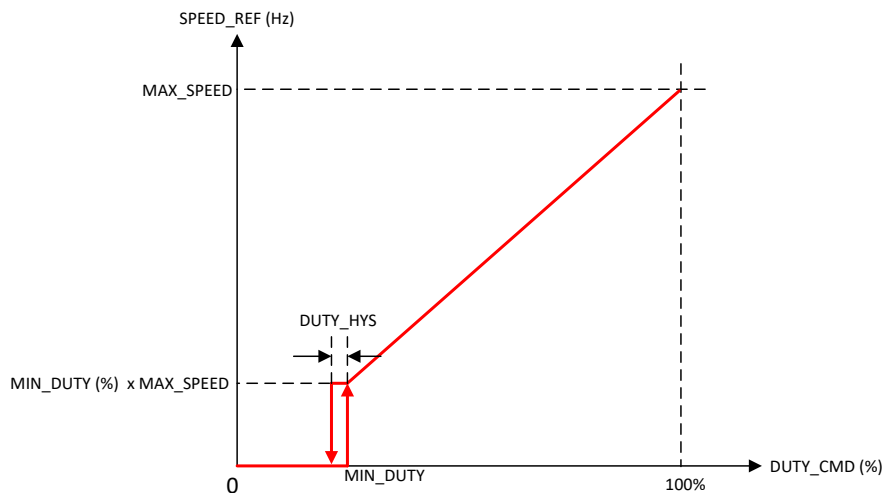
図 7-16. 速度リファレンスの伝達関数
