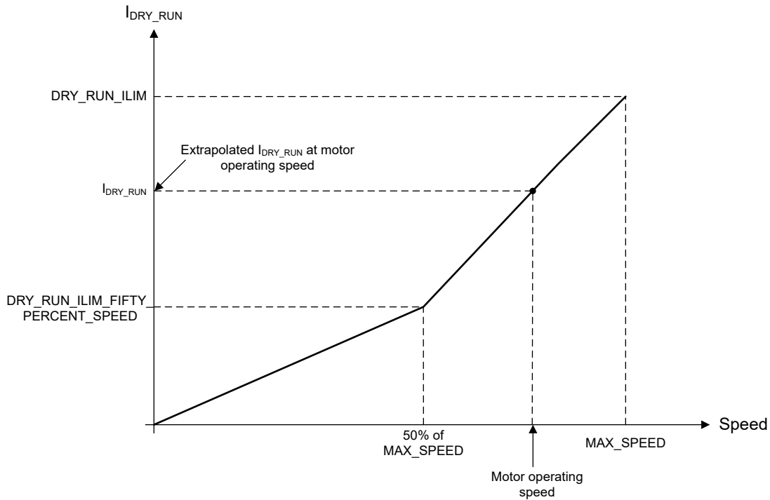
図 7-51. ドライラン検出のための可変電流スレッシュヨルド ( I_{DRY\_RUN} )
