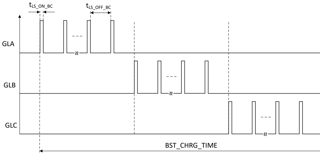
図 7-20. 起動時のブートストラップコンデンサのプリチャージ
