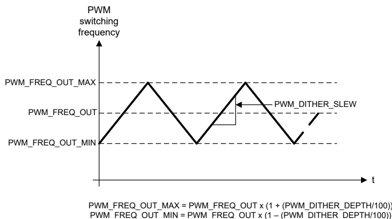
図 7-43. 三角波 PWM ディザリング
