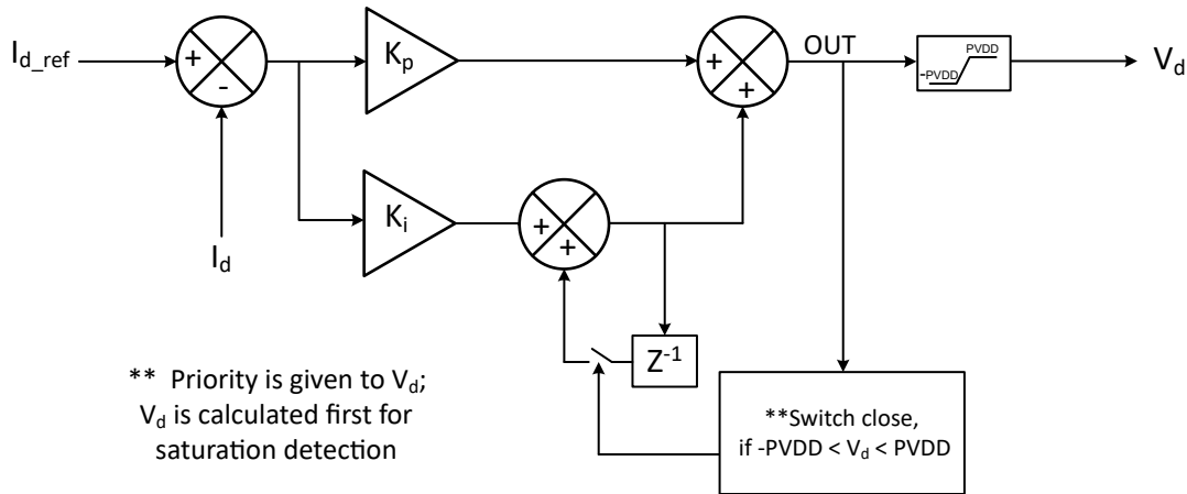
図 7-33. I_d 電流 PI 制御
