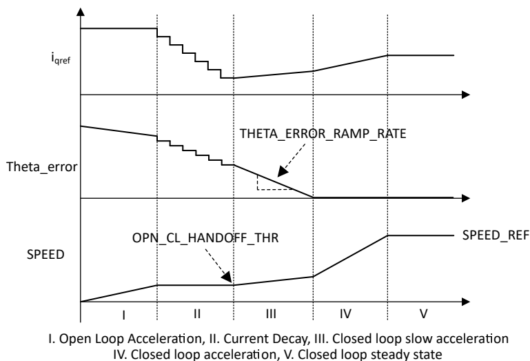
図 7-28. 開ループ - 閉ループ遷移の制御シーケンス
