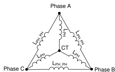
図 7-39. モーター インダクタンス
