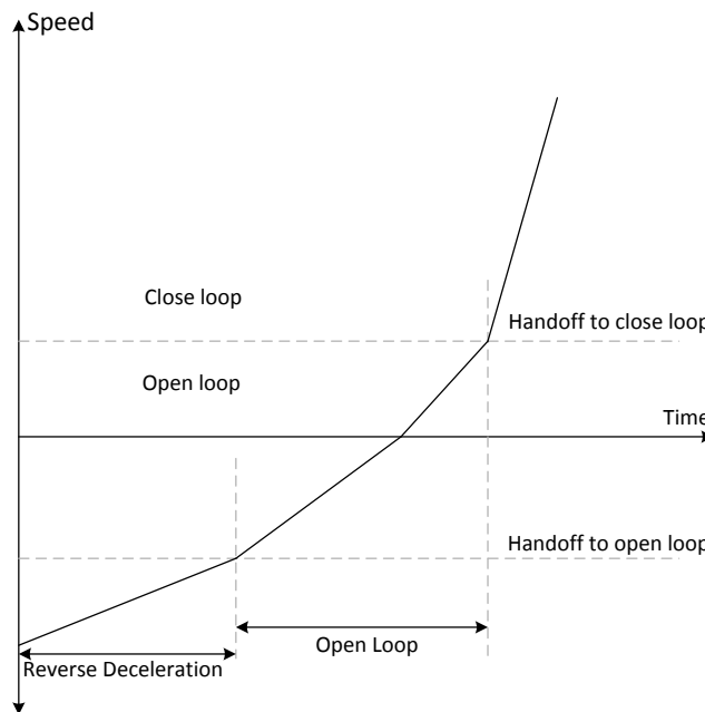
図 7-23. リバース ドライブ機能
