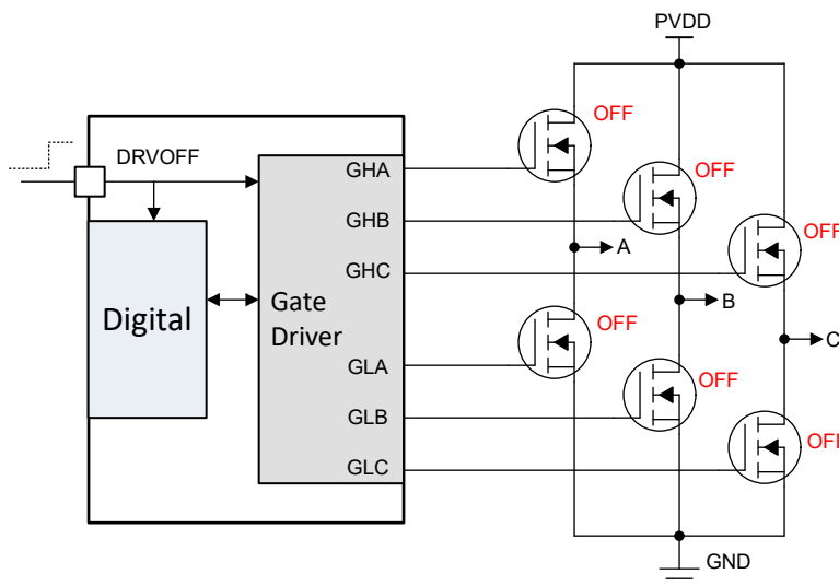
図 7-52. DRVOFF のゲート ドライバの出力状態
