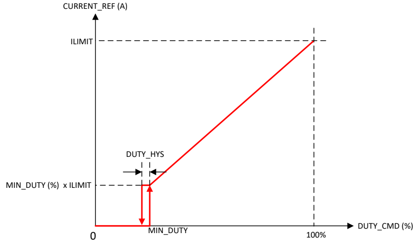
図 7-19. 電流リファレンスの伝達関数
