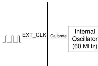
図 7-54. 外部クロック基準
