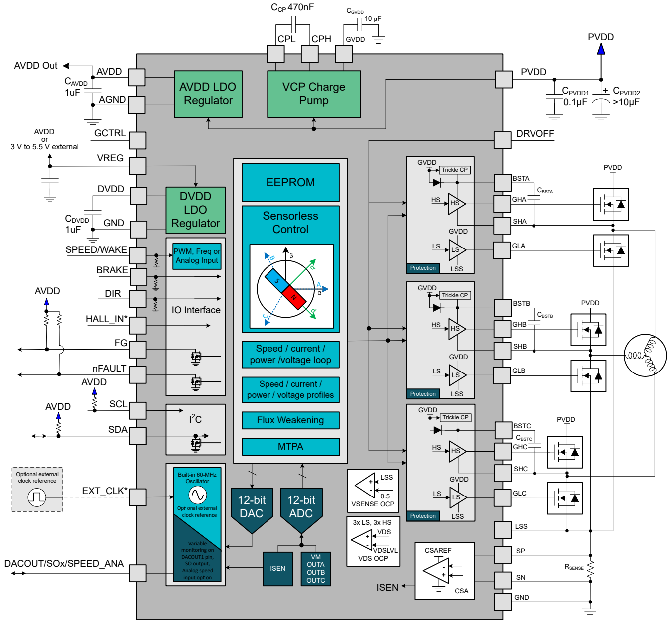
図 7-1. MCF8329HS 機能ブロック図
