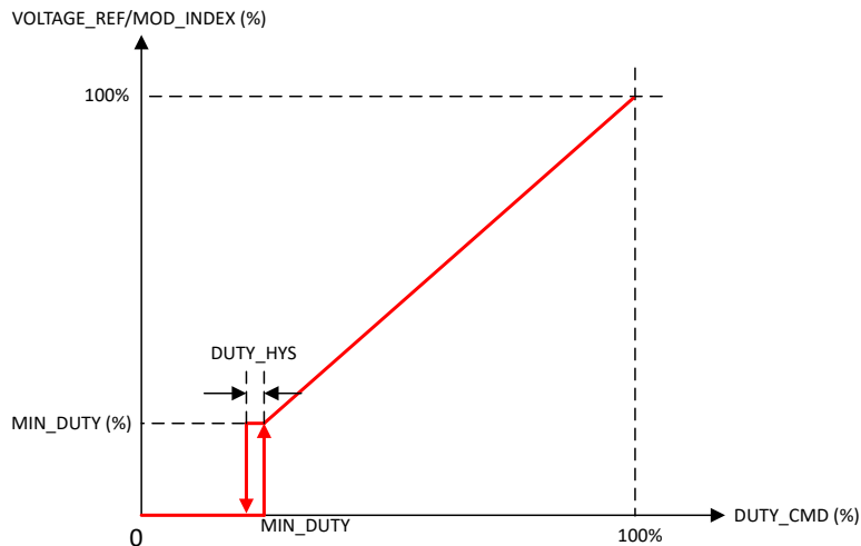
図 7-18. 電圧リファレンスの伝達関数
