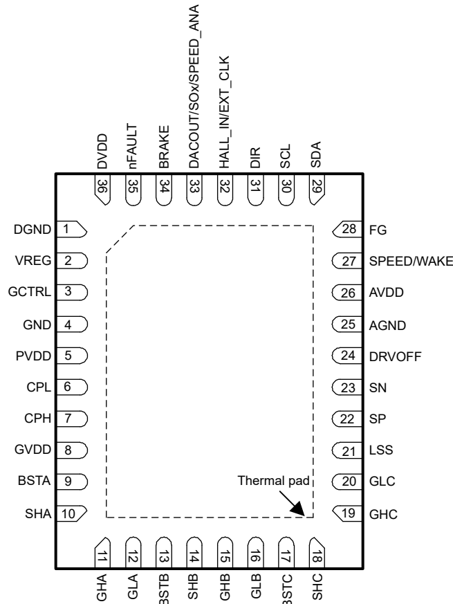
図 5-1. MCF8329HS 36 ピン WQFN (露出サーマルパッド付き) 上面図
