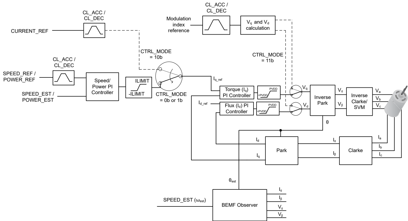
図 7-30. 閉ループ FOC 制御
