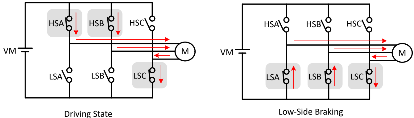
図 7-45. ローサイド ブレーキ
