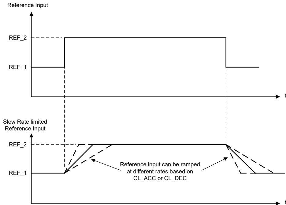
図 7-31. 閉ループ加速 / 減速スルーレート
