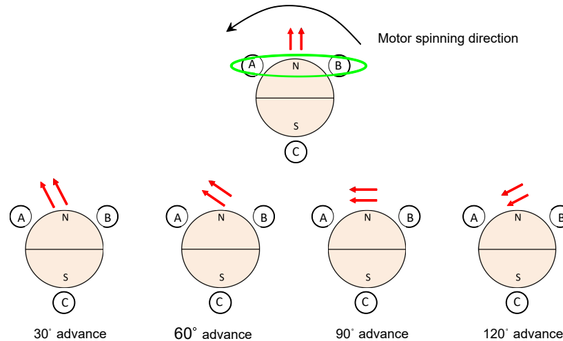
図 7-26. IPD アドバンス角度
