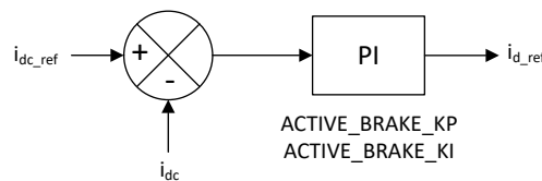
図 7-42. アクティブ ブレーキの i_{d\_ref} 電流制御ループ
