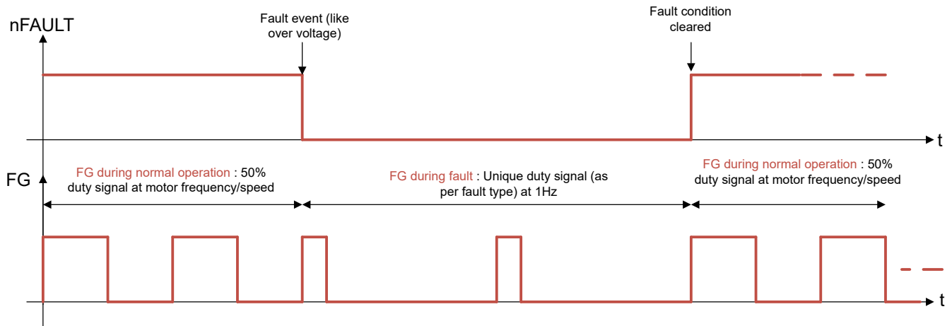
図 7-48. FG によるフォルト表示
