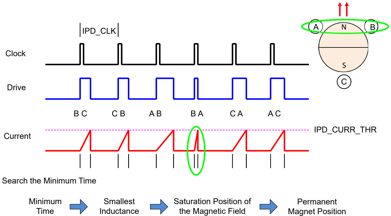
図 7-24. IPD の機能
