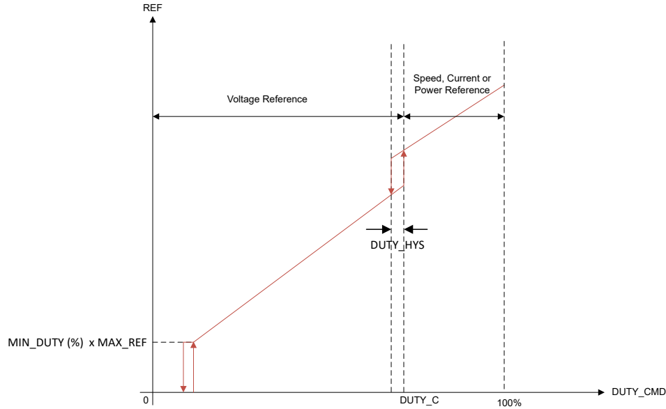
図 7-15. マルチリファレンス モード動作 (MIXED_MODE_CONFIG = 10b の場合)
