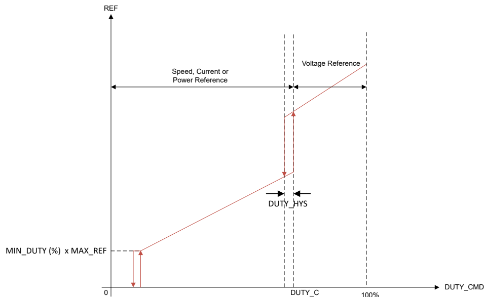
図 7-14. マルチリファレンス モード動作 (MIXED_MODE_CONFIG = 01b の場合)
