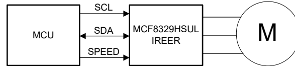
図 10-5. MCF8329HSULIREER を搭載した IEC 60730 機能安全システム
