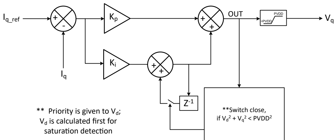
図 7-34. I_q 電流 PI 制御
