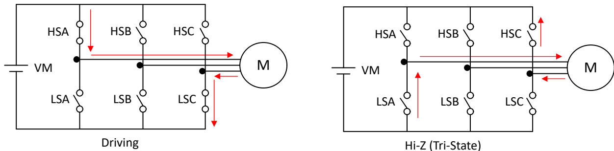
図 7-25. IPD 解放ハイ インピーダンス モード
