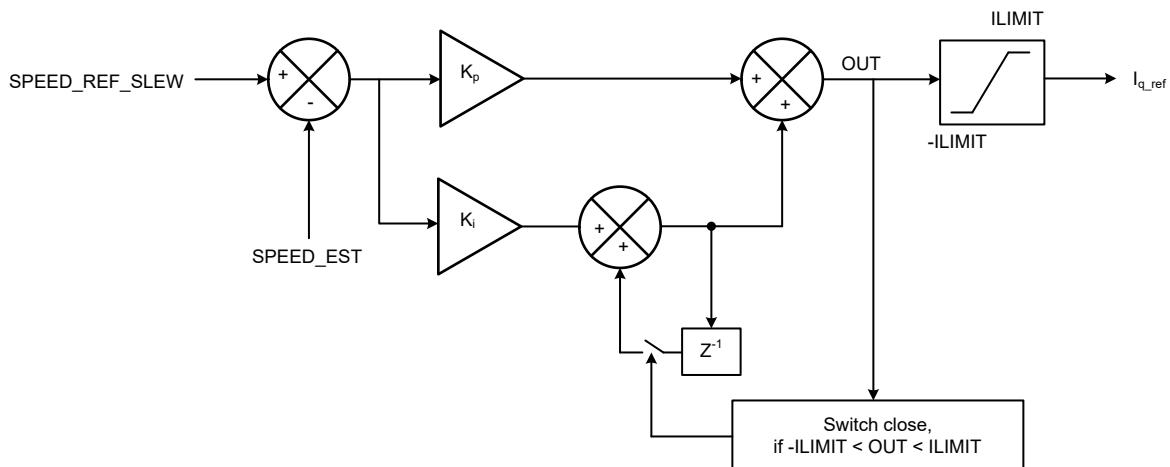
図 7-32. 速度 PI 制御
