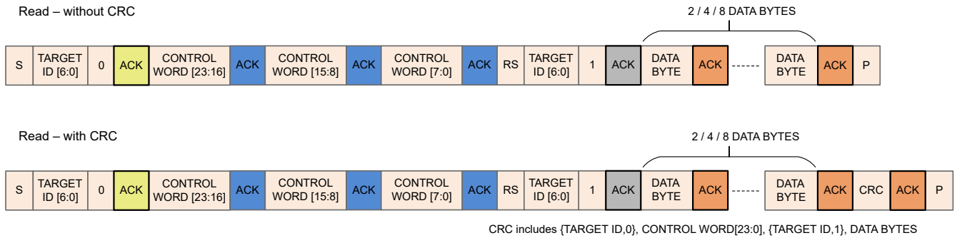
図 7-56. I 2 C 読み出しトランザクションシーケンス
