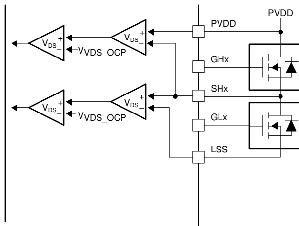
図 7-49. VDS モニタ
