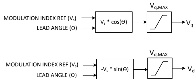
図 7-36. 開ループ電圧制御
