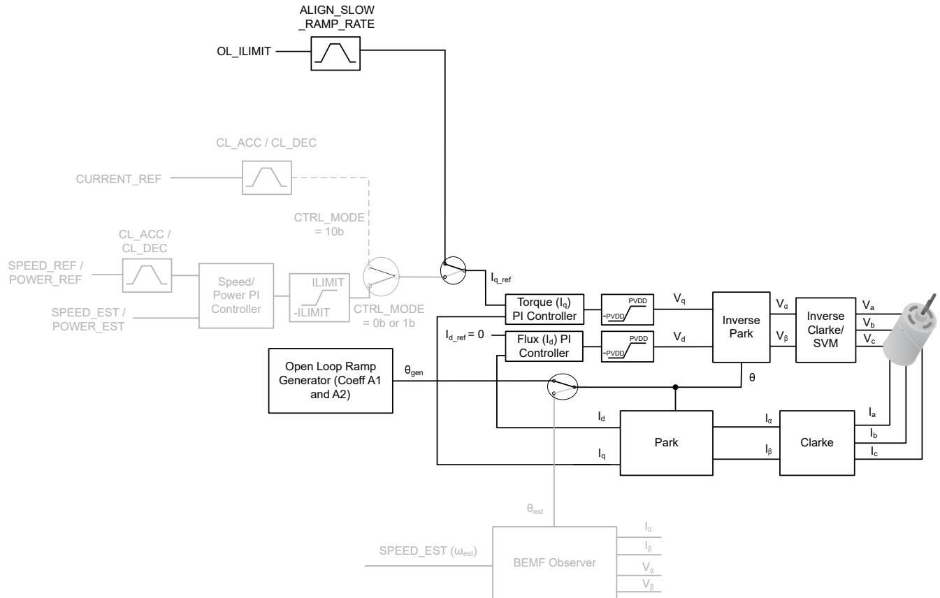
図 7-27. 開ループ
