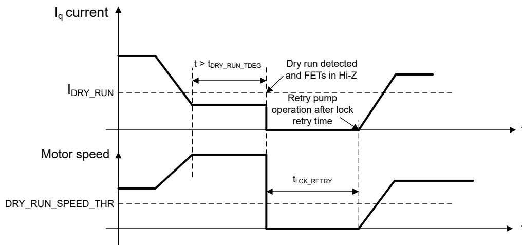
図 7-50. ドライ ラン検出
