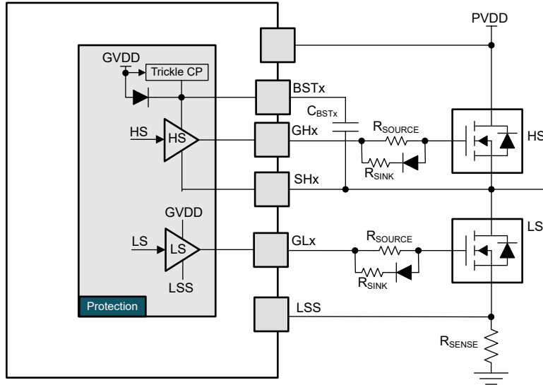
図 10-3. ゲート ドライバ出力 (別個ソースおよびシンク電流経路を使用)
