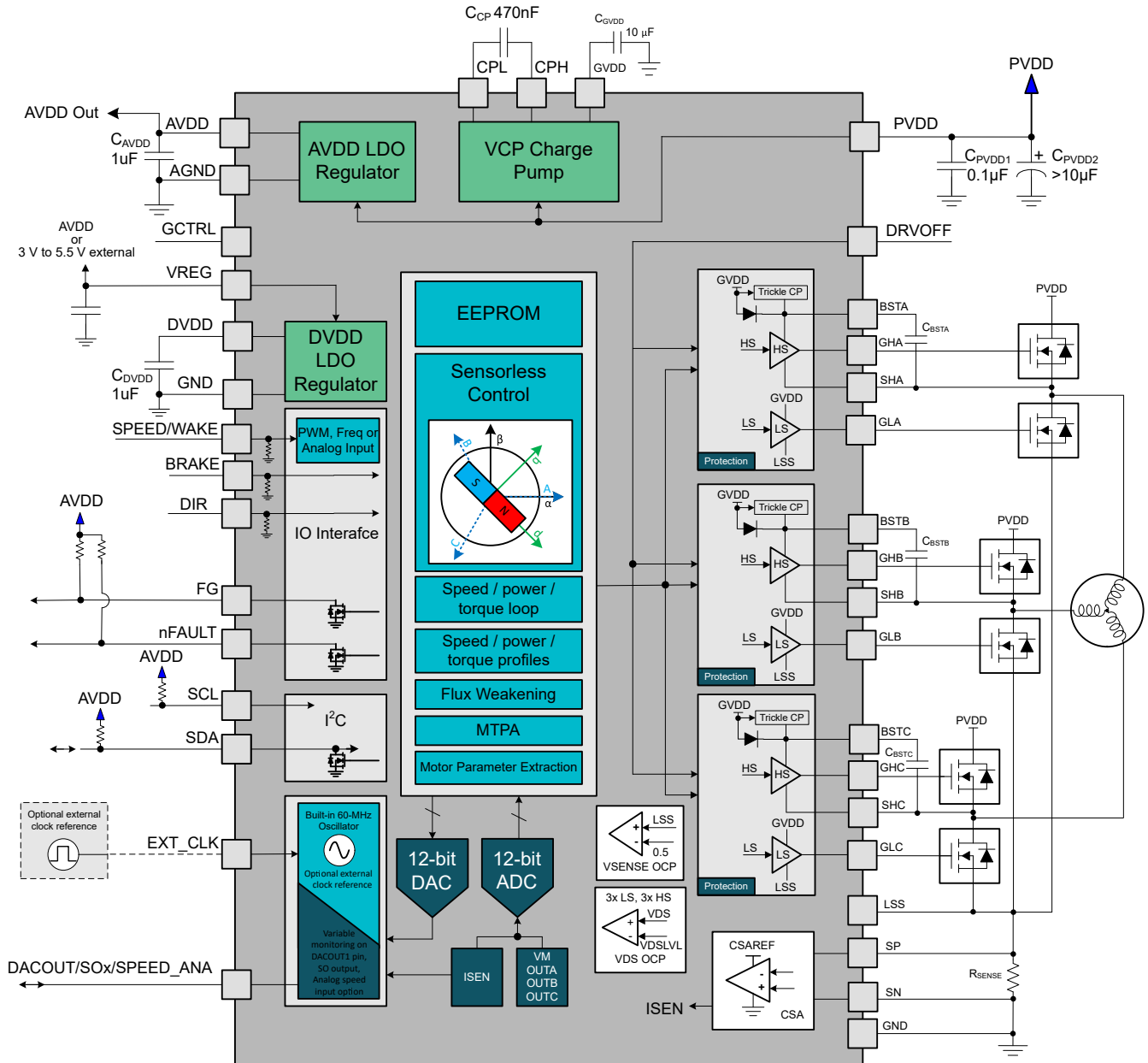
図 10-1. MCF8329HS の代表的な回路図
