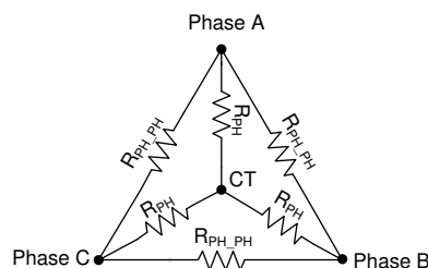
図 7-38. モータ抵抗
