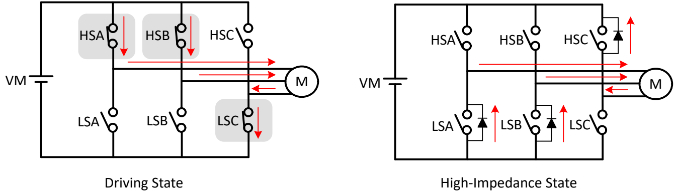
図 7-44. コースト (ハイ インピーダンス) モード
