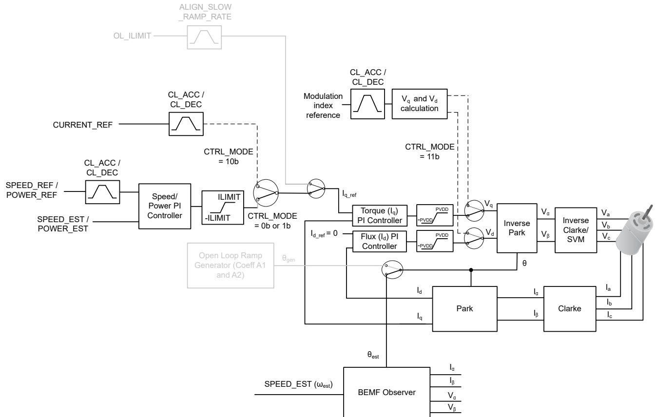
図 7-29. 開ループから閉ループへの遷移
