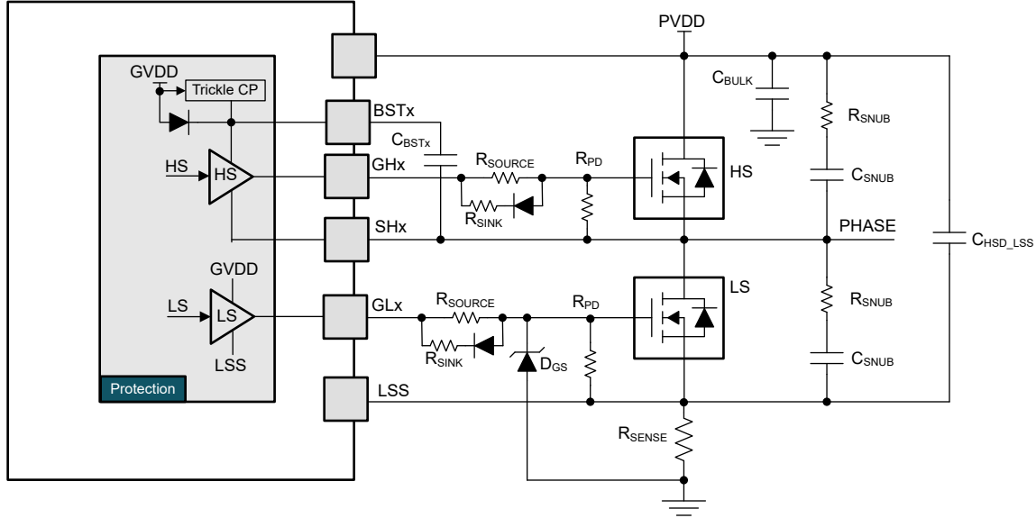
図 10-4. 任意の外部出力段部品
