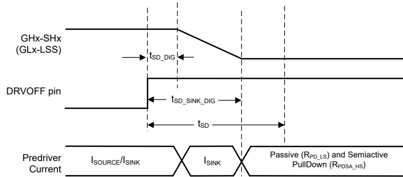
図 7-53. ゲートドライバシャットダウンシーケンス
