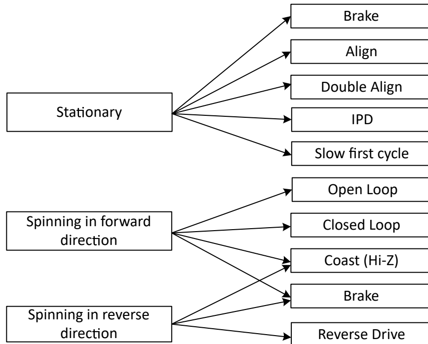
図 7-21. 異なる初期条件でのモーターの起動
