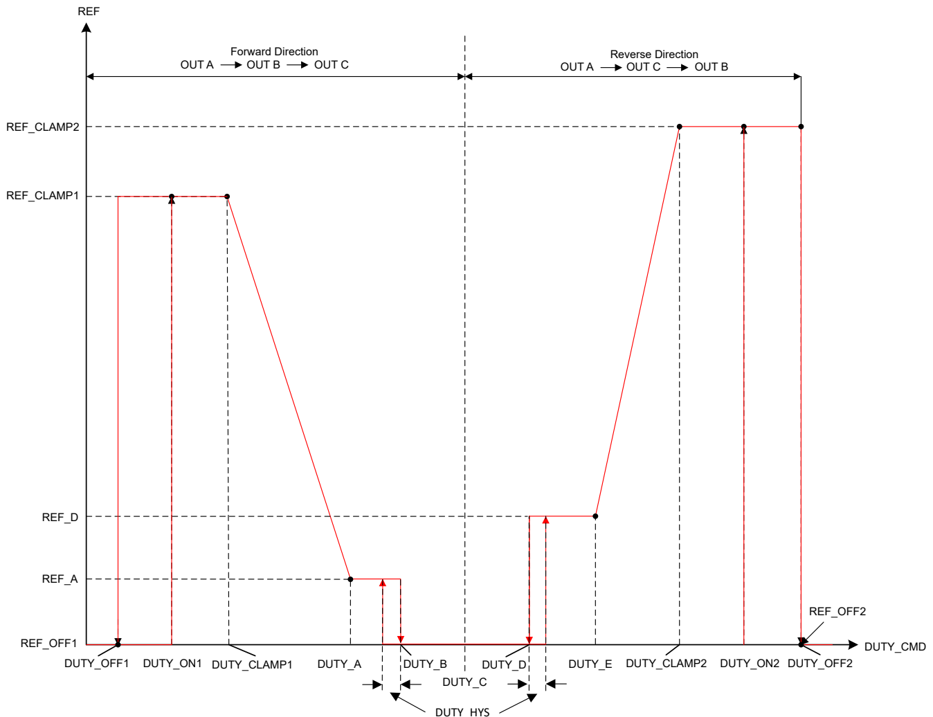
図 7-13. 双方向制御プロファイル
