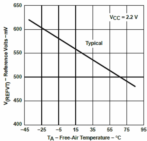
図 20. 温度対 V_{(REFVT)} , V_{CC} = 2.2V
