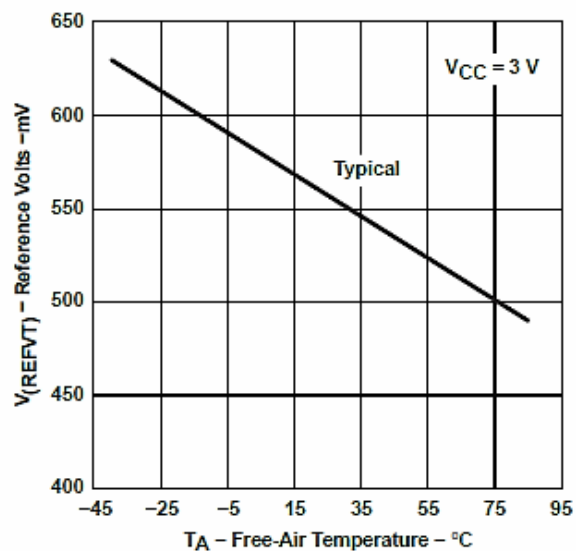
図 19. 温度対 V_{(REFVT)} , V_{CC} = 3V
