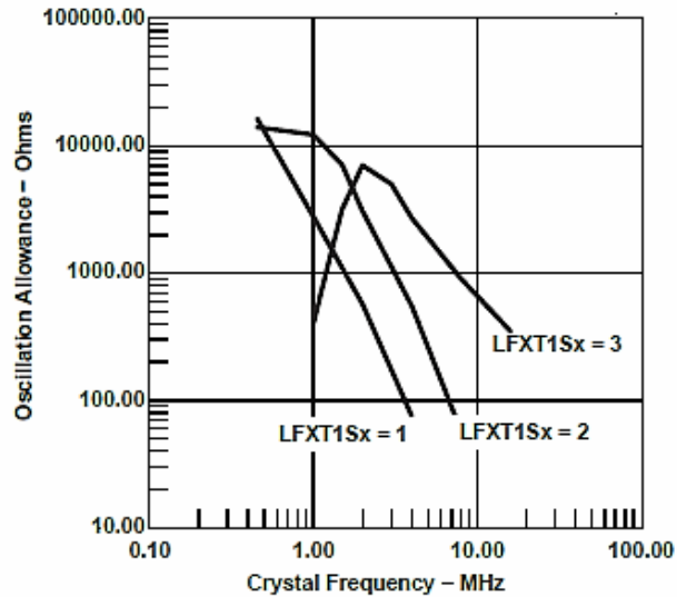
図 14. クリスタル周波数対発振許容値、 C_{L,eff} = 15 \text{ pF} , T_A = 25^\circ\text{C}
