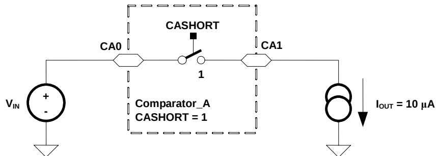
図 18. コンパレータ_A+ 短絡抵抗測定条件
