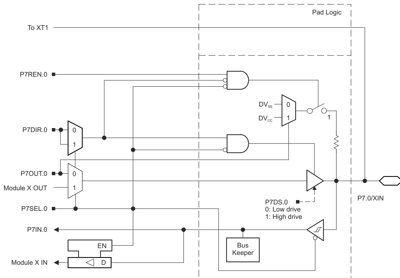
9-11. Port P7 (P7.0) Diagram
