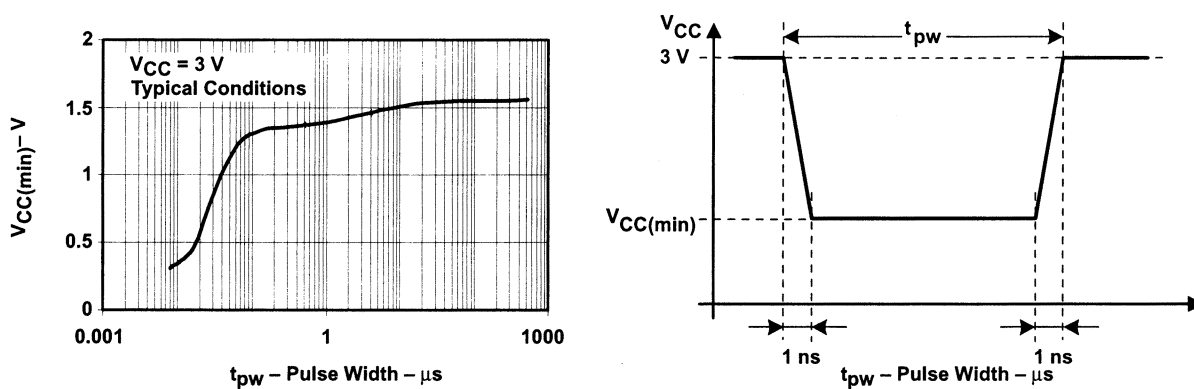
図 11. POR/ブラウンアウト信号を生成するための VCC(min) レベル (矩形波電圧降下)
