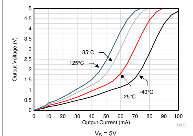
図 5-35. 出力電圧スイングと出力電流との関係 (シンク) (新しいダイ)
