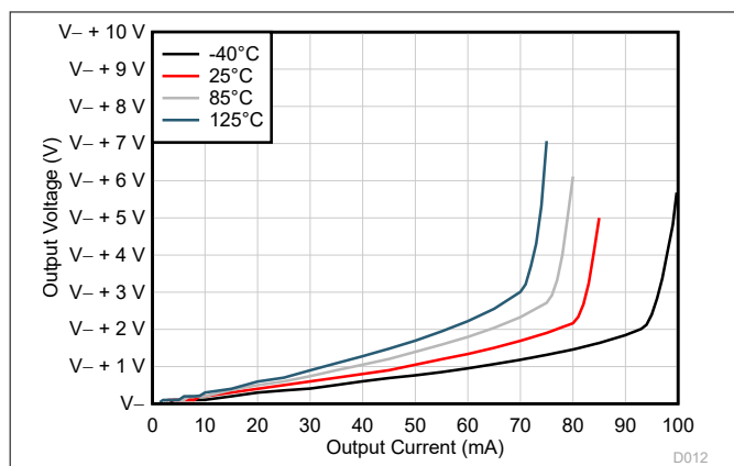
図 5-33. 出力電圧スイングと出力電流との関係 (シンク) (新しいダイ)
