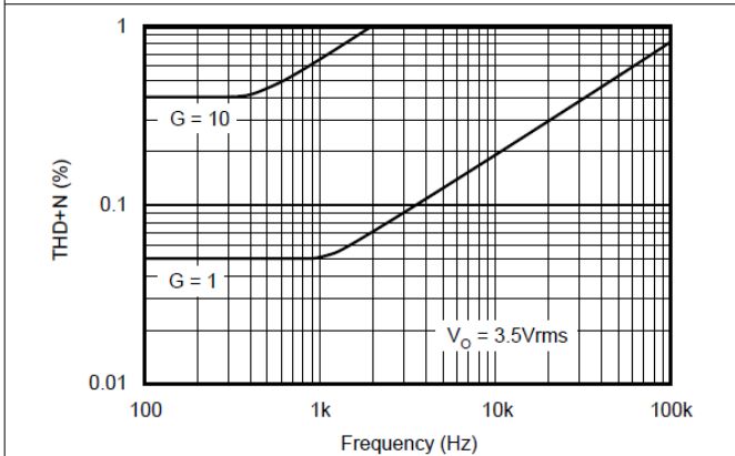
図 5-7. 全高調歪 + ノイズと周波数との関係 (古いダイ)
