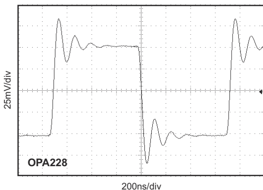
図 8-6. 小信号ステップ応答、 G = 2 、 C_{LOAD} = 100\text{pF} 、 入力信号=50mVp-p
