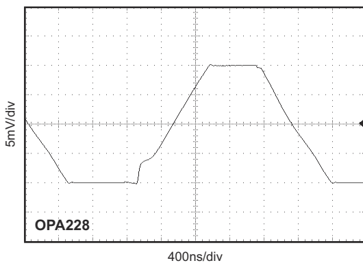
図 8-4. 大信号ステップ応答、 G = 2 、 C_{LOAD} = 100\text{pF} 、 入力信号=5Vp-p
