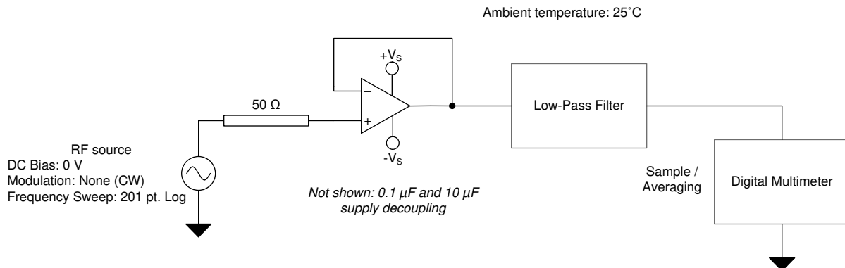
図 7-9. EMIRR IN+ のテスト構成の回路図
