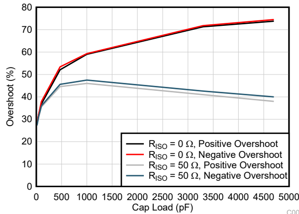
図 6-5. 小信号オーバーシュートと容量性負荷との関係 (出力ステップ 10mV、 G = 1 )
