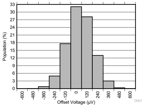
15462 個のアンプにおける分布、 T_A = 25^\circ\text{C}
