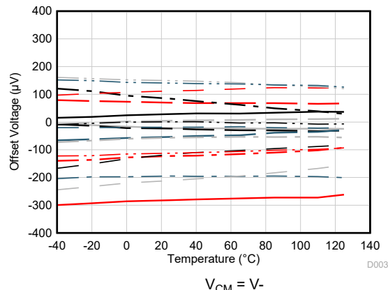
図 5-4. オフセット電圧と温度との関係
