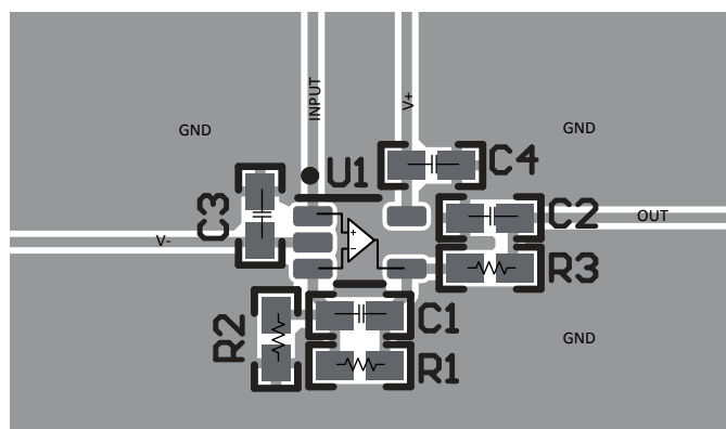
図 7-4. SC70 (DCK) パッケージのレイアウト例
