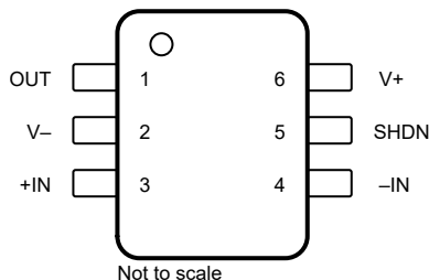
図 4-3. OPA991S-Q1 DBV パッケージ、 6 ピン SOT-23 (上面図)
