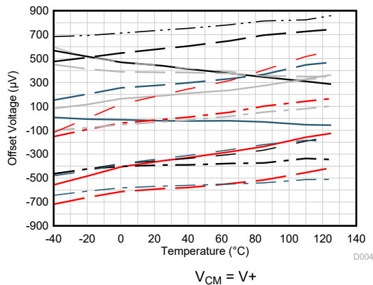
図 5-3. オフセット電圧と温度との関係
