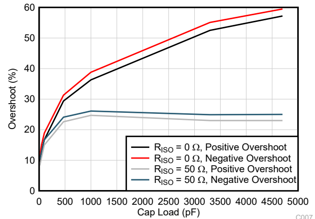
図 6-6. 小信号オーバーシュートと容量性負荷との関係 (出力ステップ 10mV、 G = -1 )
