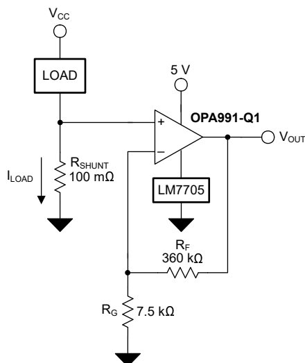
図 7-1. ローサイド電流センシング・アプリケーションの OPAx991-Q1
