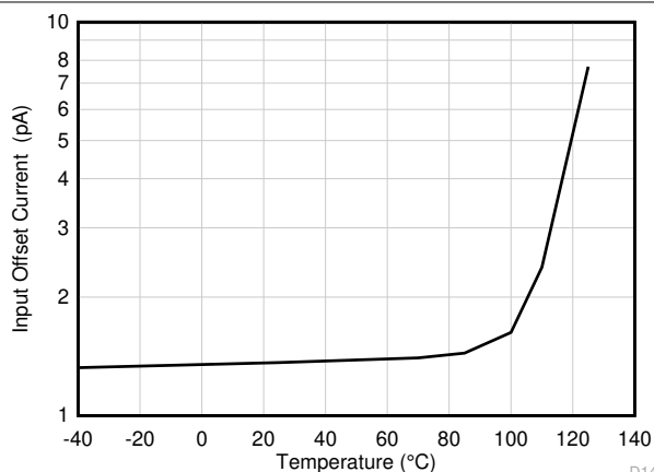
図 6-14. I_{OS} vs 温度
