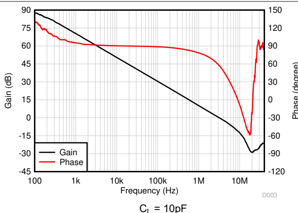
図 6-18. 開ループゲインおよび位相と周波数との関係
