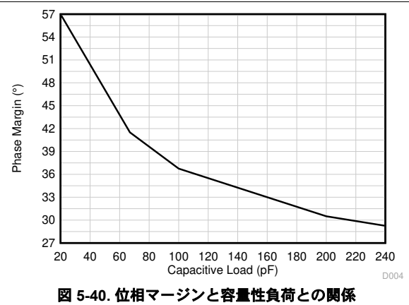
図 5-40. 位相マージンと容量性負荷との関係
