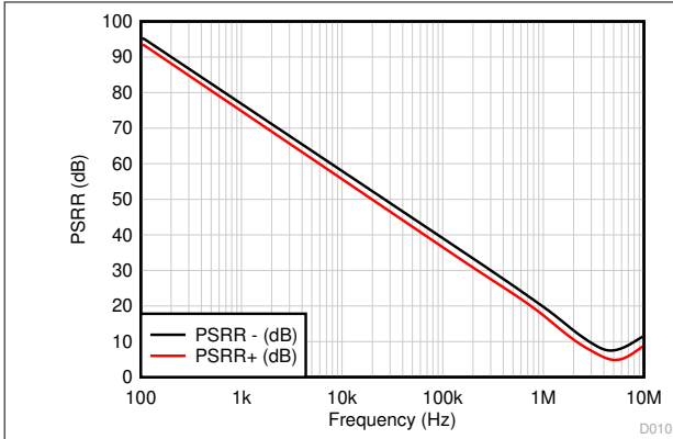
図 5-25. PSRR と周波数との関係
