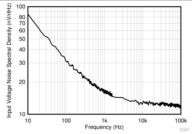
図 5-30. 入力電圧ノイズスペクトル密度
