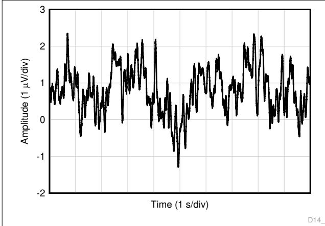
図 5-29. 時間領域での 0.1Hz~10Hz の電圧ノイズ
