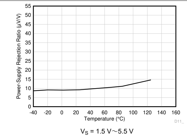
図 5-26. DC PSRR と温度との関係
