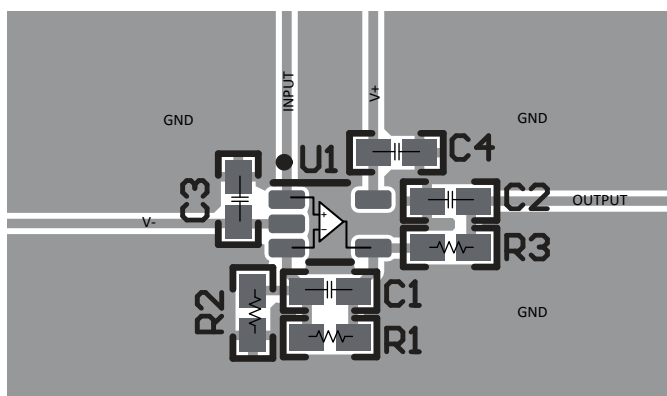
図 7-4. 非反転構成用オペアンプの基板レイアウト - SC70 (DCK) パッケージ
