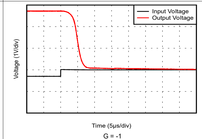
図 5-34. 過負荷回復
