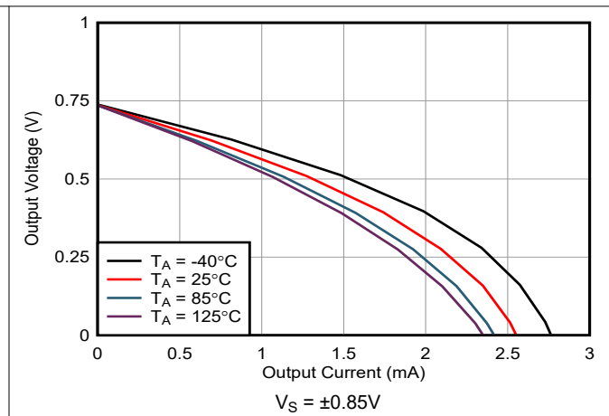
図 5-26. 出力電圧と出力電流との関係 (ソース)
