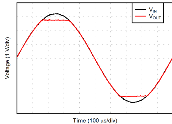
図 6-32. 位相反転が発生しない
