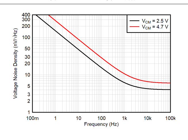
図 6-22. 電圧ノイズと周波数との関係
