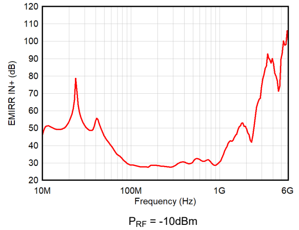
図 6-40. EMIRR と周波数との関係
